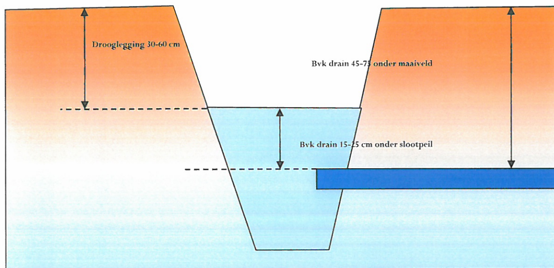
Illustratie van aanlegseisen onderwaterdrainage
