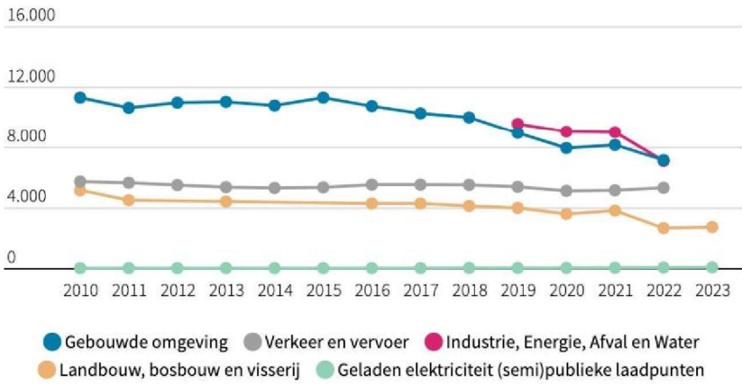
CO 2 -uitstoot energieverbruik sectoren Zuid-Holland, kton
