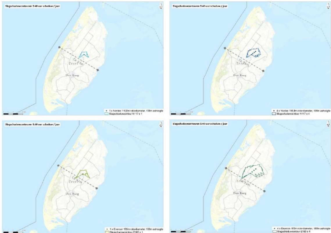
Abbeelding 8.13 Indicatieve slagschaduwcontour (boven: 3,6 MW turbine, onder: 5,6 MW turbine)
