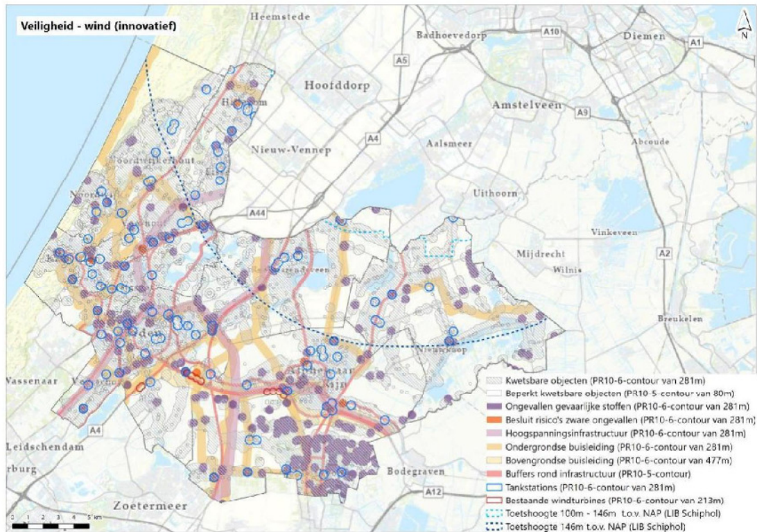
Abbeelding 7.21 Veiligheidsafstanden voor een innovatieve windturbine
