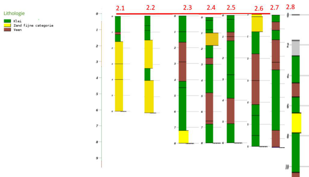
Figuur 3.7b Gegevens bodemopbouw profiel 2.1 t/m 2.8
