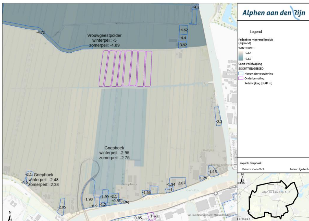
Figuur 3.10 Polderpeilen en peilafwijkingen in de Gnephoekpolder.
