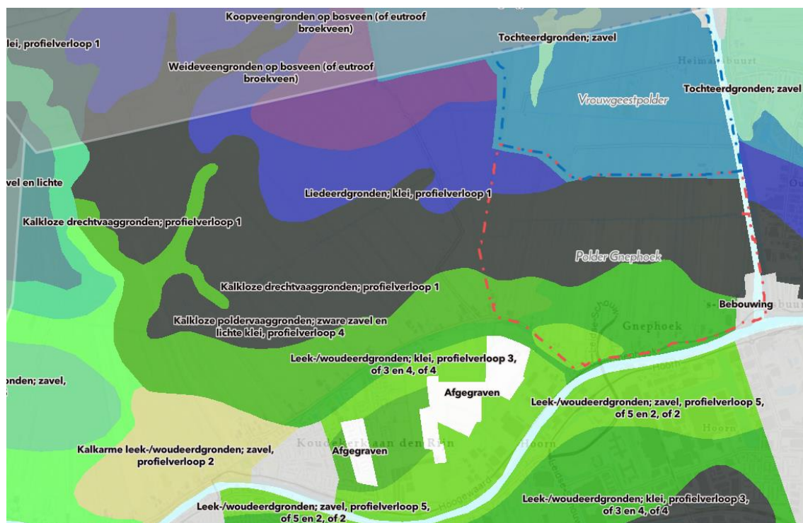
Figuur 3.4 Bodemsoorten Gnephoekpolder
