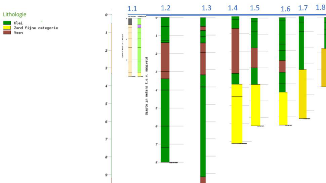
Figuur 3.6b Gegevens bodemopbouw profiel 1.1 t/m 1.7
