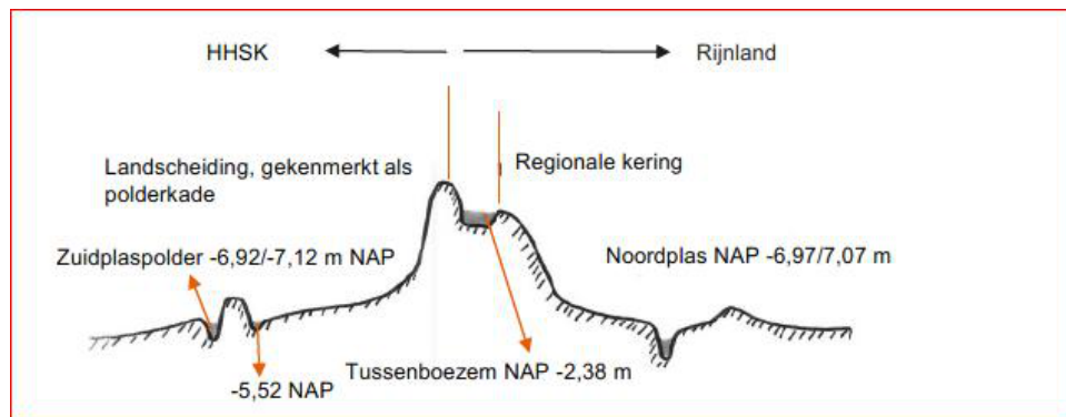
Figuur 7: regionale waterkering Kleikade in het deelgebied Provinciale wegden (Arcadis, 2018)
