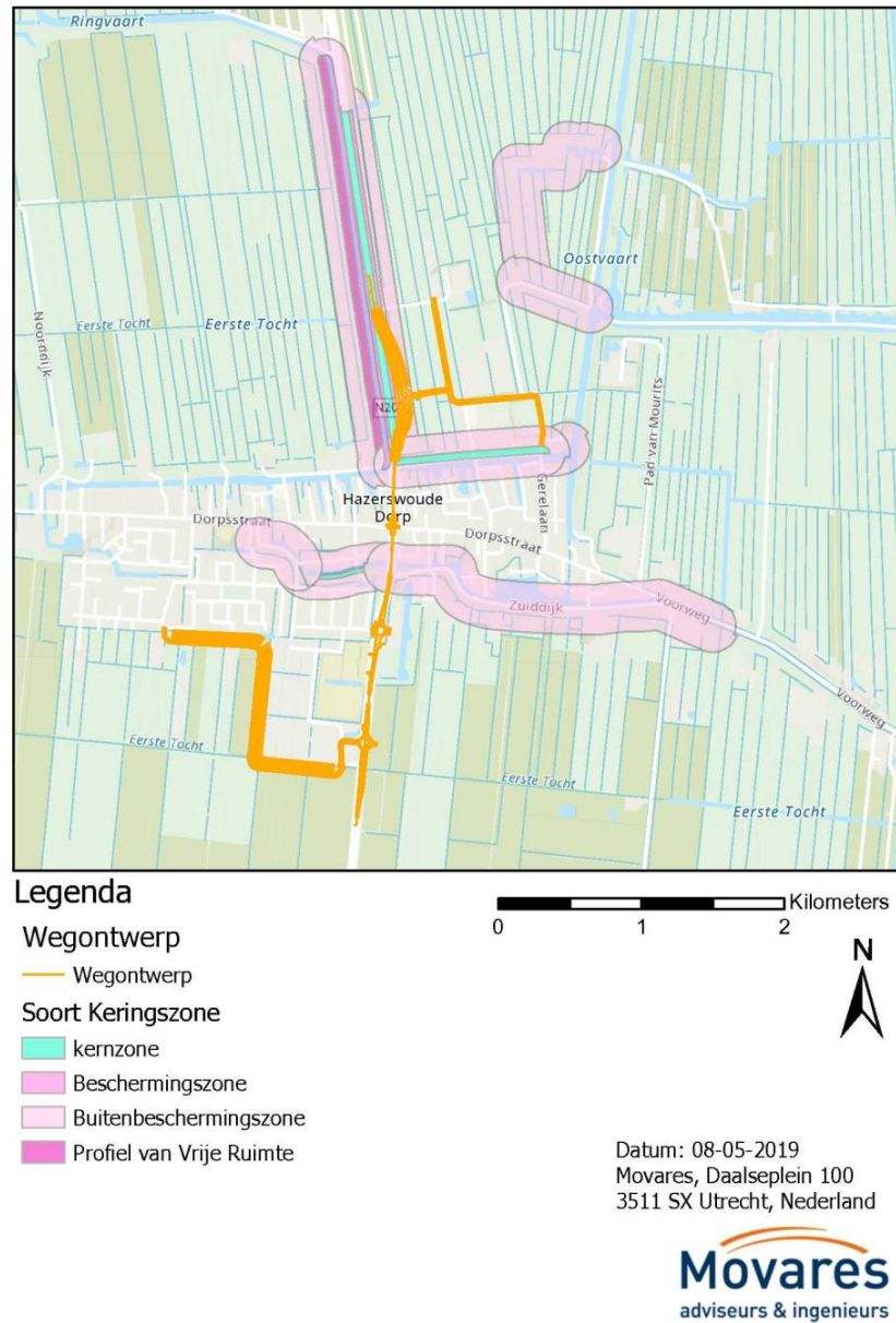
Figuur 8: regionale waterkeringen in alle deelgebieden in Hazerswoude-Dorp, ter indicatie is X-Robuust weergegeven.
