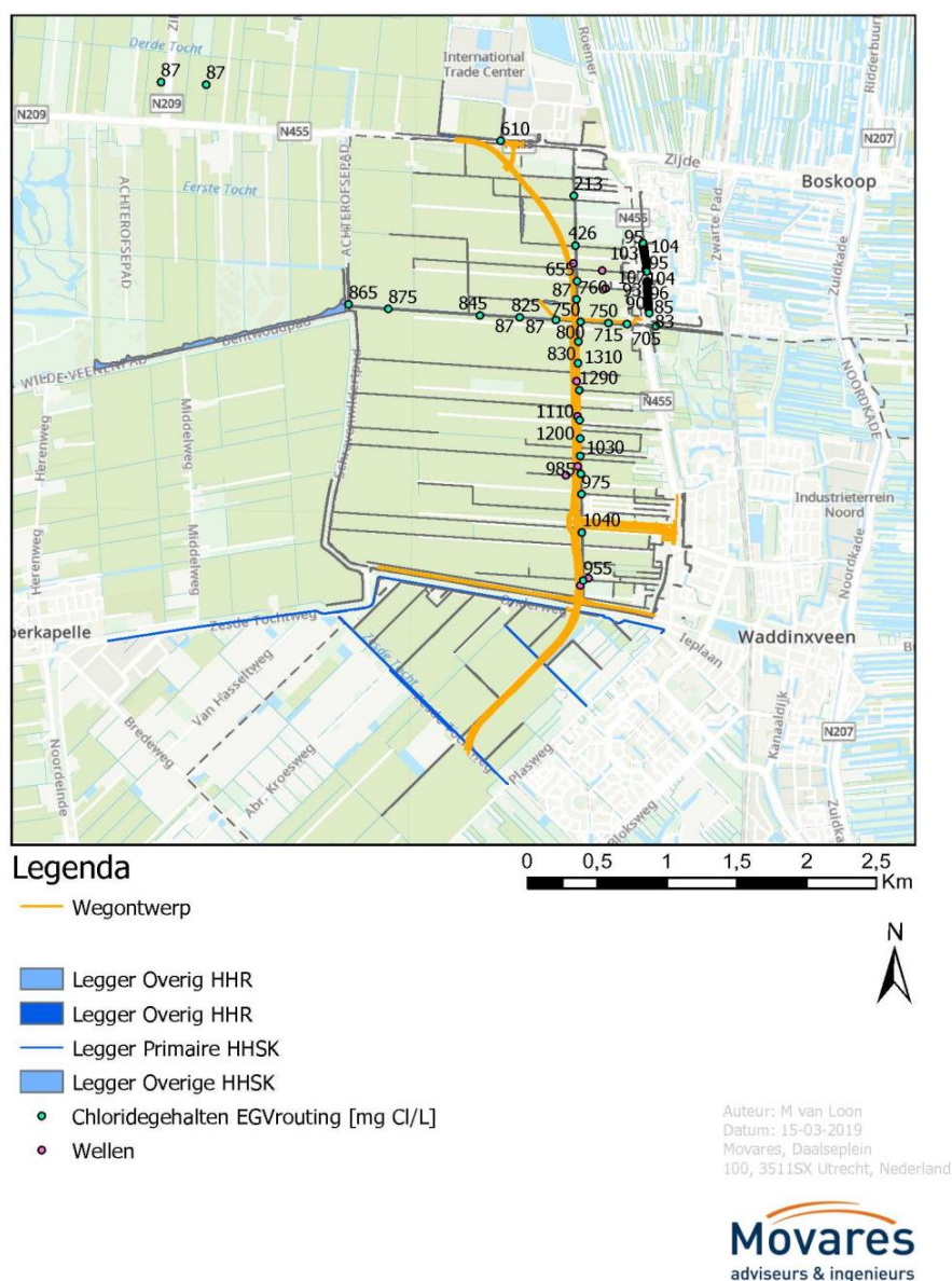
Figuur 15: wellen en chloridengehalten in het deelgebied Provinciale wegdelen
