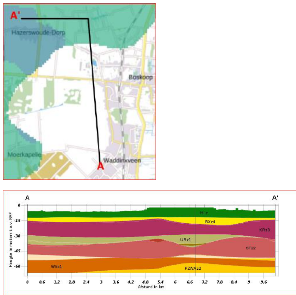
Figuur 11: traject en bodemopbouw over de 4 deelgebieden (Dinoloket, 2019)
