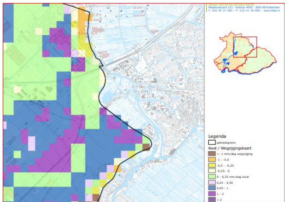
Figuur 13: kwelgebieden in polders (Arcadis, 2016)
