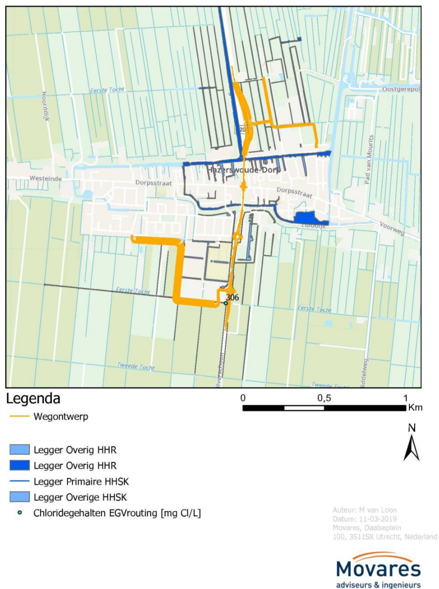
Figuur 18: chloridgehalten in alle deelgebieden in Hazerswoude-Dorp, ter indicatie is X-Robuust weergegeven
