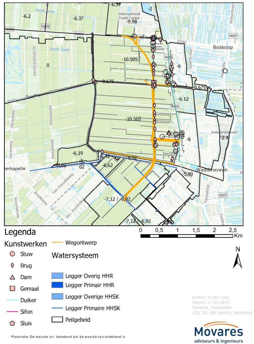
Figuur 9: watersysteem in het deelgebied Provinciale wegdelen
