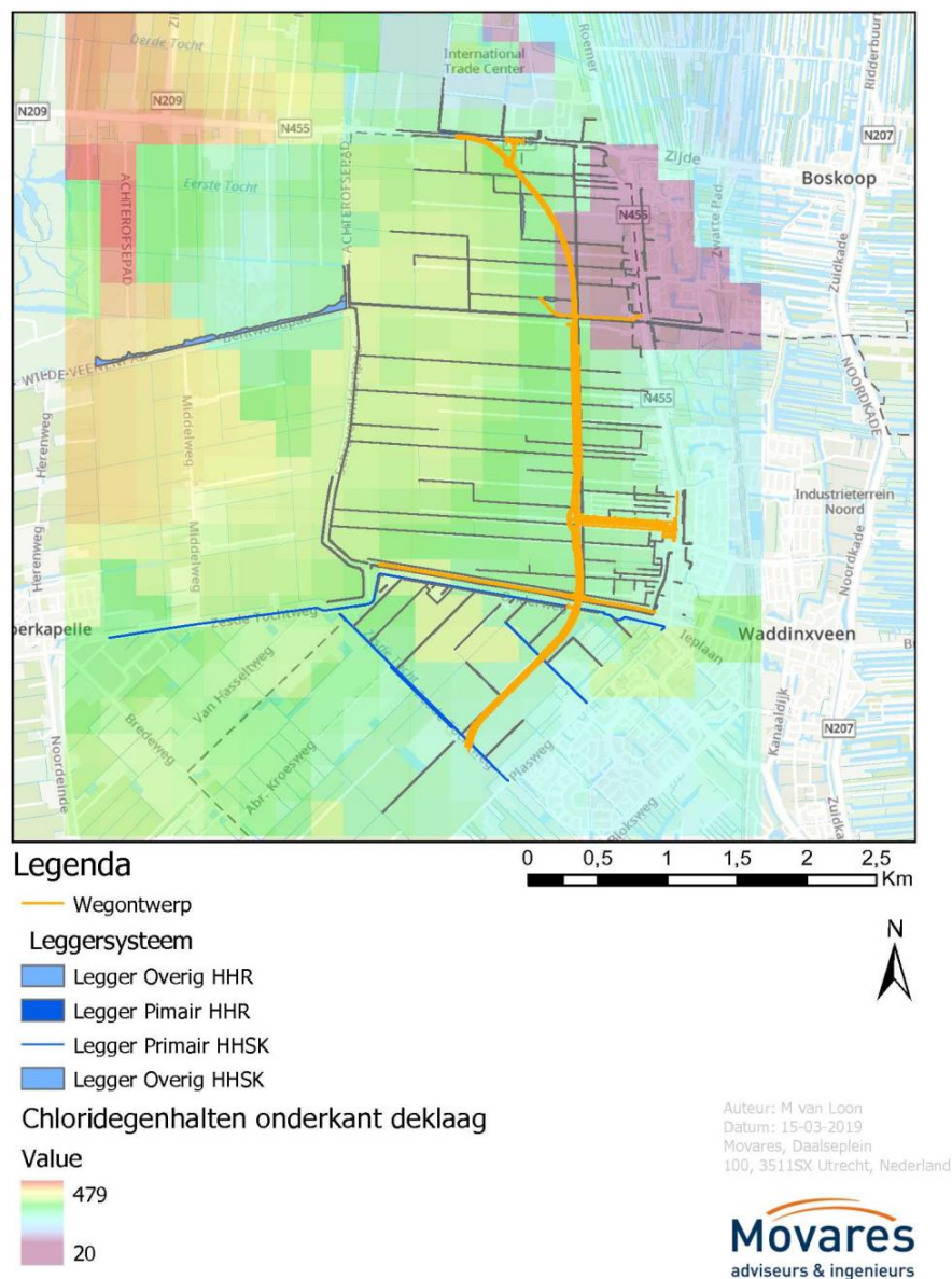
Figuur 20: chloridengehalten [mg Cl/l] onderkant deklaag in het deelgebied Provinciale wegdelen
