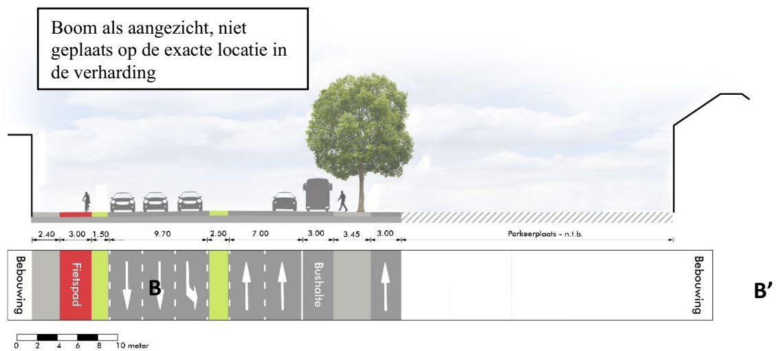
Figuur 13: Doorsnede Hazerswoude-Dorp Dorpsstraat B-B'
