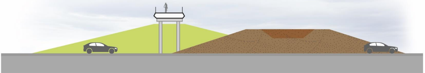
Figuur 22: Doorsnede Kleikade en fietsbrug, aanzicht vanaf de weg (doorsnede H)
