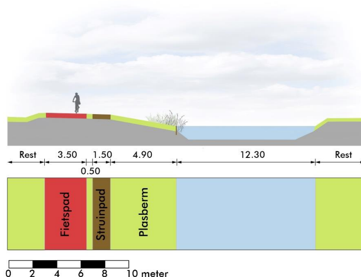
Figuur 16: Doorsnede fietspad langs de Maaltocht (doorsnede E)
