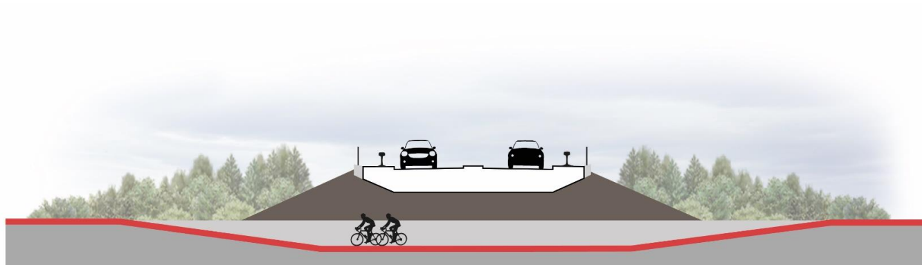
Figuur 17: Doorsnede Maaltocht (doorsnede C)
