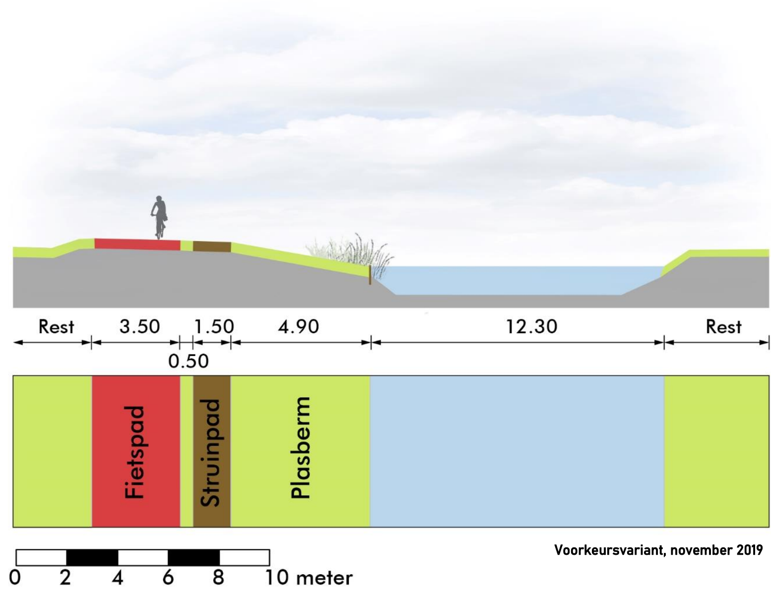
Doorsnede fiets- en voetpad Maaltoch (E)
