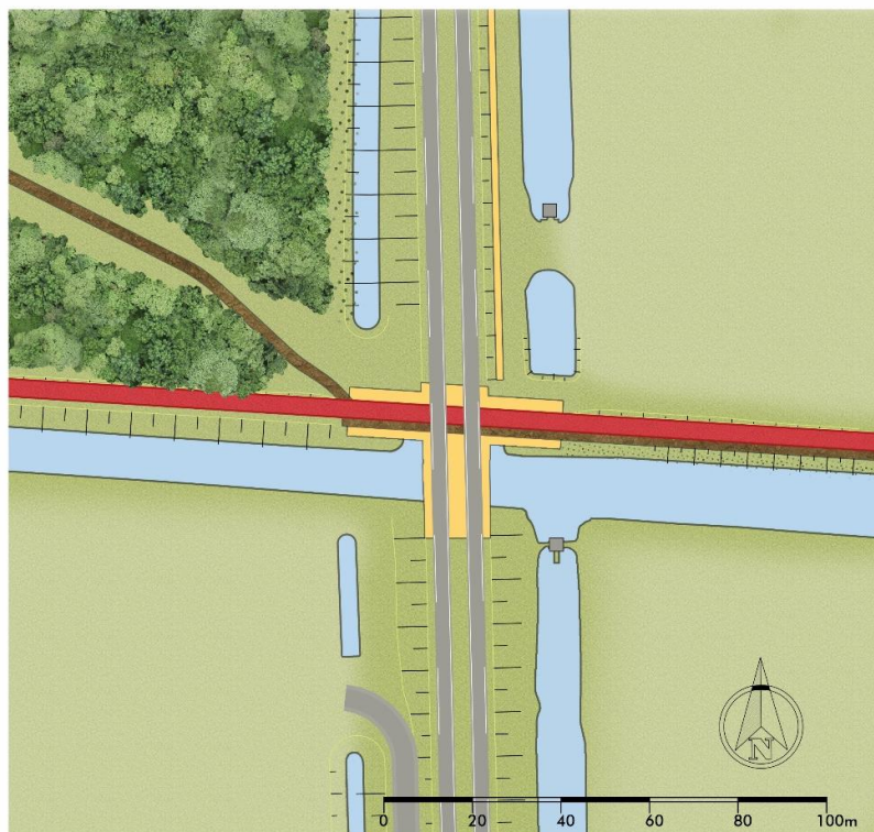
Figuur 15: Plattegrond kunstwerk ter hoogte van Maaltocht (detail 4)
