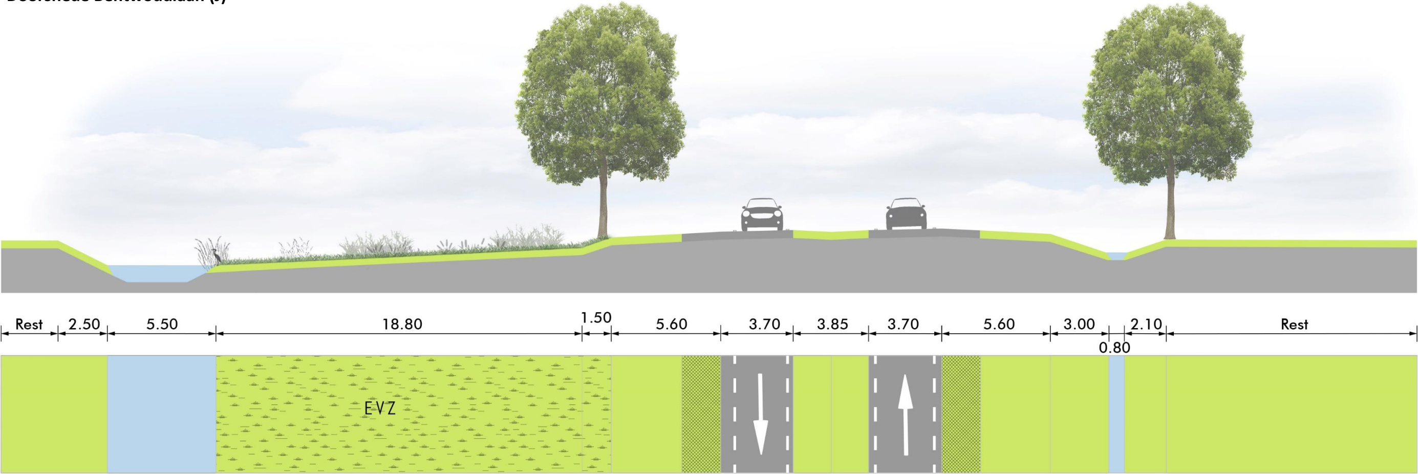
Doorsnede Bentwoudlaan (J)
