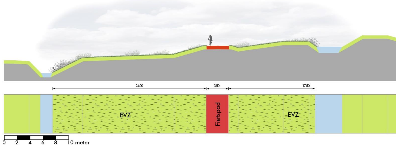
Figuur 25: Doorsnede van de kleikade met hierop de EVZ en het fietspad (doorsnede I)
