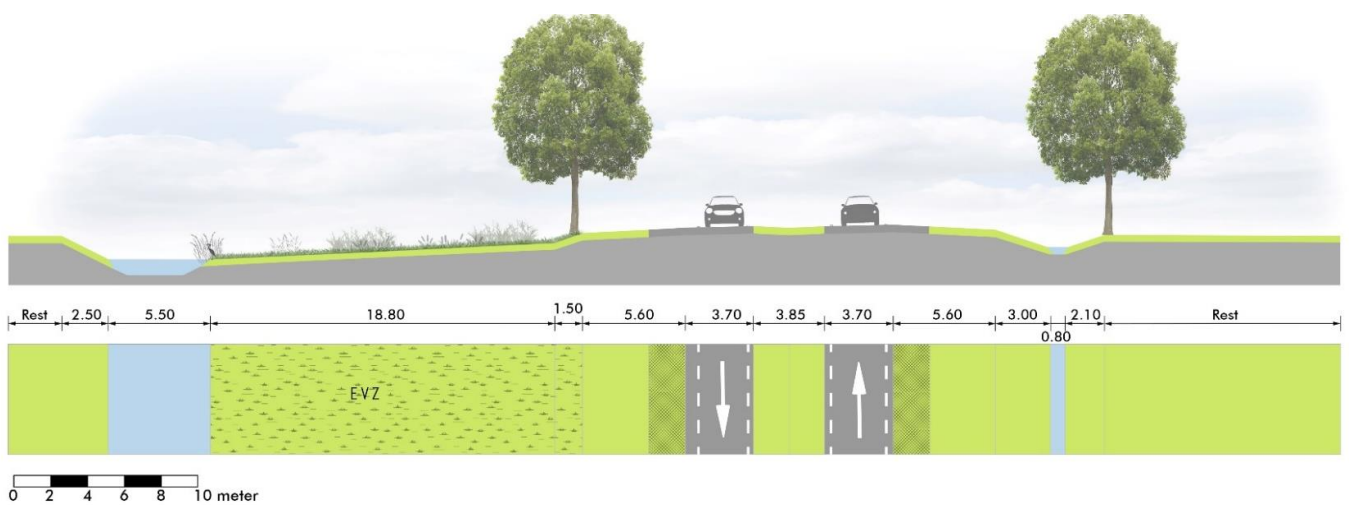
Figuur 23: Doorsnede van de weg met aan de westzijde de EVZ (doorsnede J)
