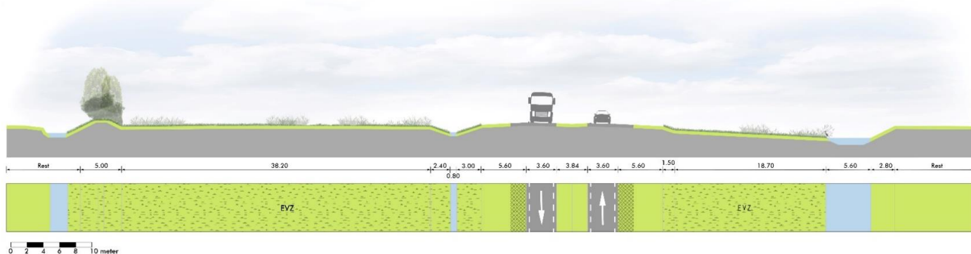
Figuur 24: Doorsnede van de weg met aan beide zijden de EVZ (doorsnede K)
