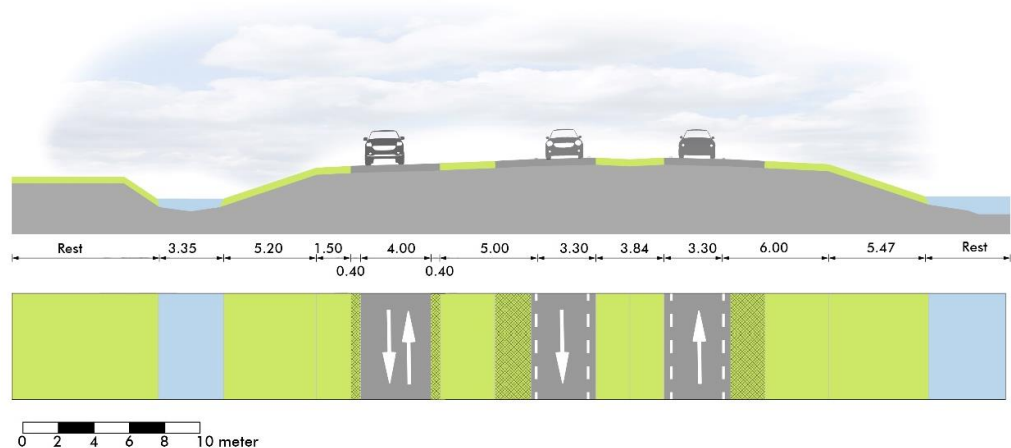
Figuur 19: Doorsnede Verlengde Bentwoudlaan tussen het Bentwoud en de Kleikade (doorsnede F)
