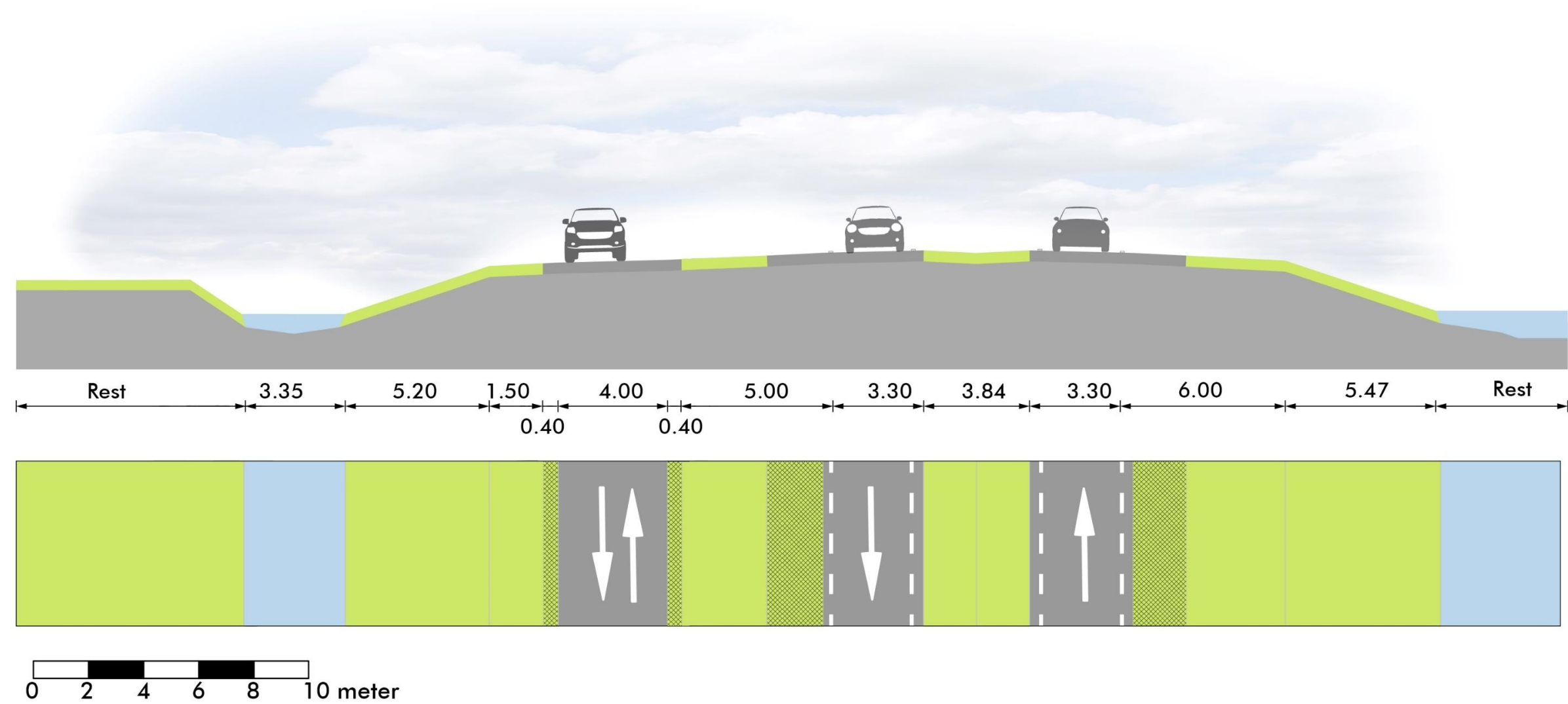
Doorsnede verlengde Bentwoudlaan (F)
