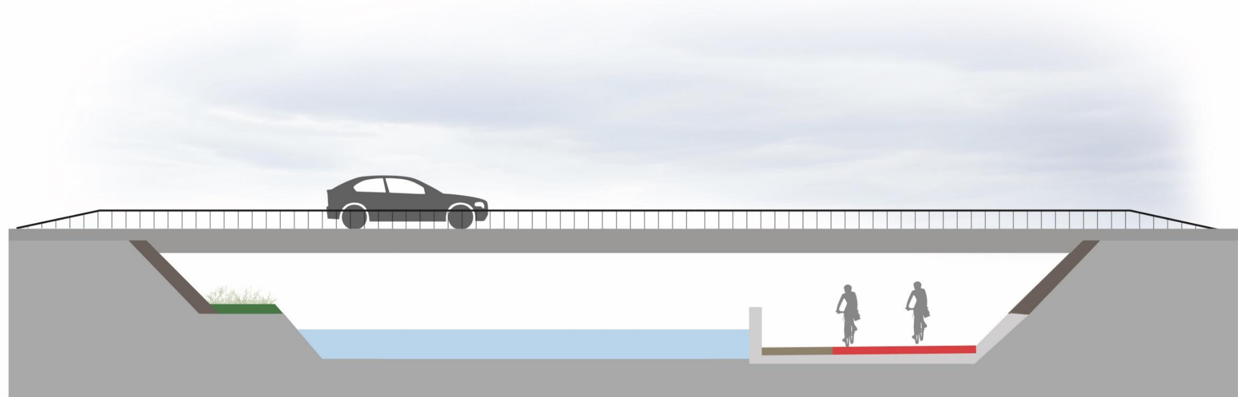
Doorsnede kunstwerk onderdoorgang Maaltocht, naar westen kijkend (D)
