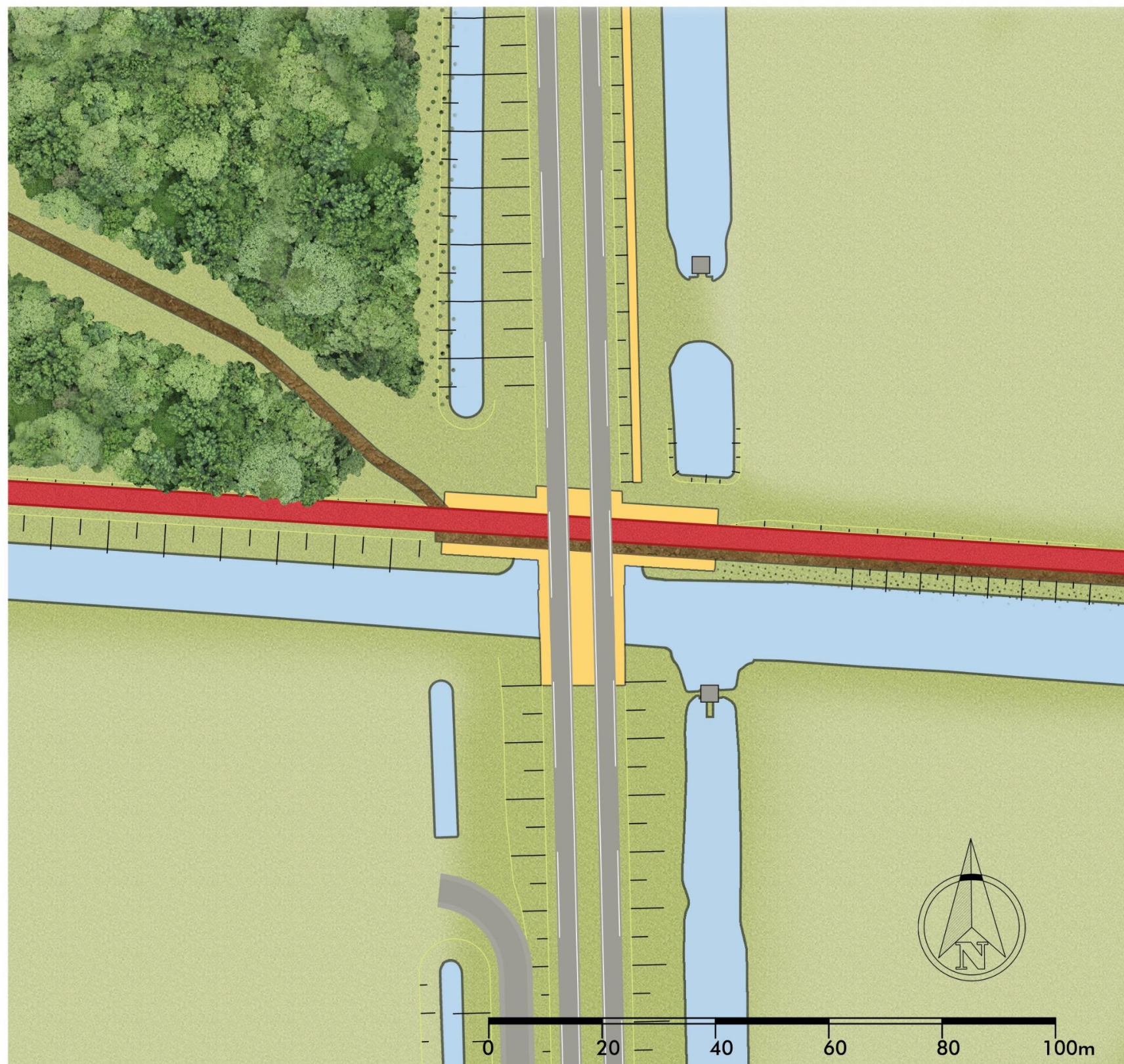
Detail 4 Onderdoorgang Maaltocht Voorkeursvariant, november 2019
