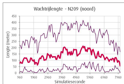
Figuur 29: Wachtrijlengte op de noordtak van de rotonde gedurende de avondspits
