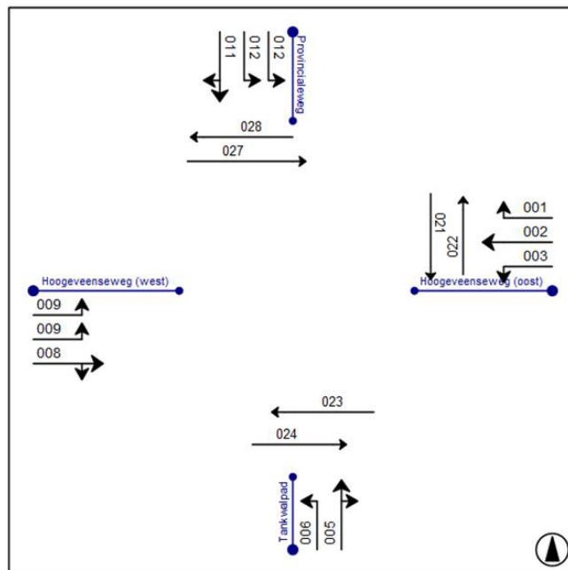
Figuur 38: De minimale kruispuntconfiguratie voor kruispunt 6
