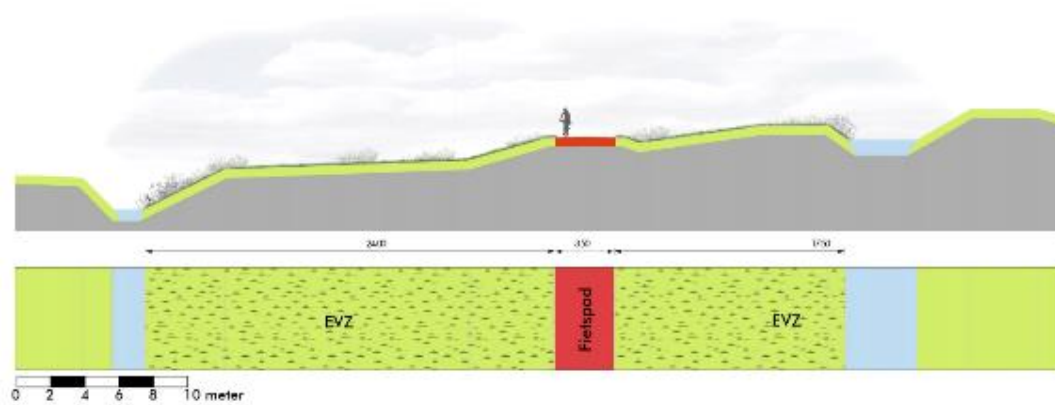
Figuur 3.17 Profiel EVZ langs de Kleikade
