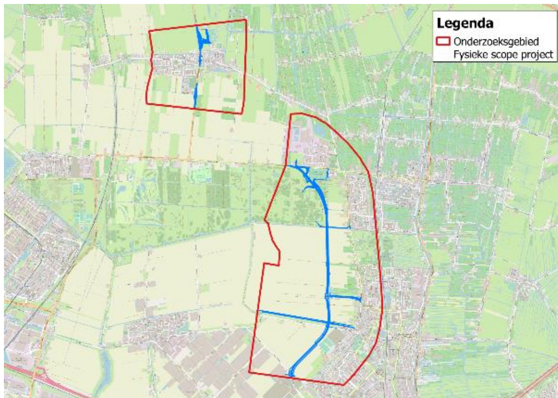
Figuur 7.3 Onderzoeksgebied trillingsonderzoek (Bron: trillingsonderzoek)
