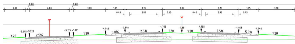
Figuur 21: doorsnede 7 Verlengde Bentwoudlaan met Boerenpad metrerings 2400.000
