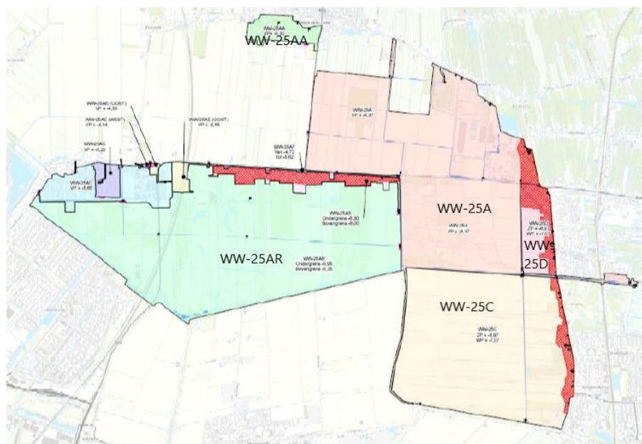
Figuur 16: Indeling toekomstige peilvakken (Toelichting bij peilbesluit en voorstel maatregelen, 2018 Rijnland)
