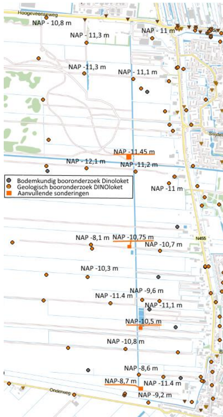
Figuur 11: diepte onderkant zandlaag
