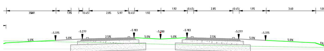
Figuur 22: doorsnede 10 Verlengde Bentwoudlaan metrerings 4250.000
