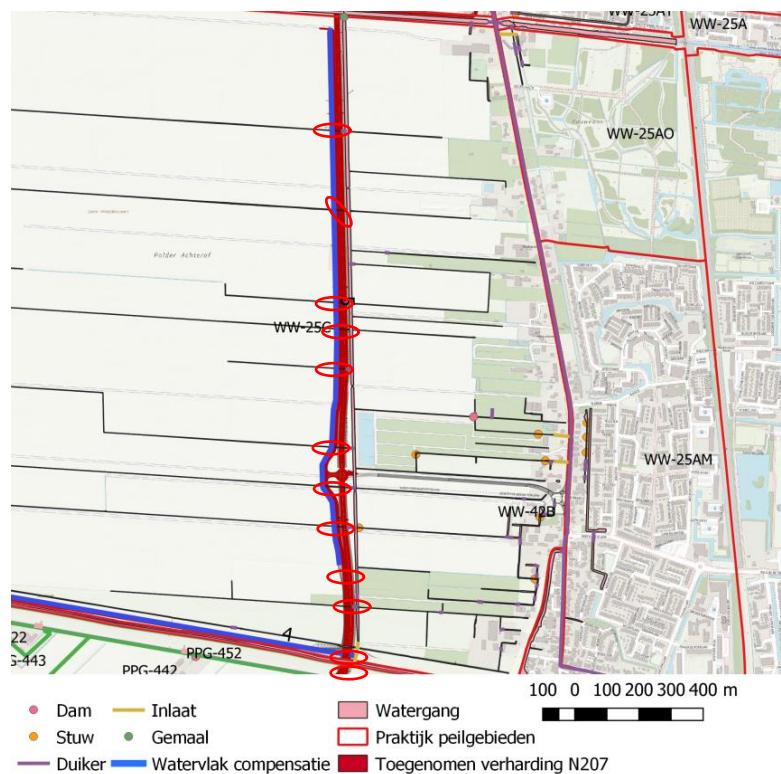
Figuur 23: overzicht verharding en watergangen verlengde Bentwoudlaan
