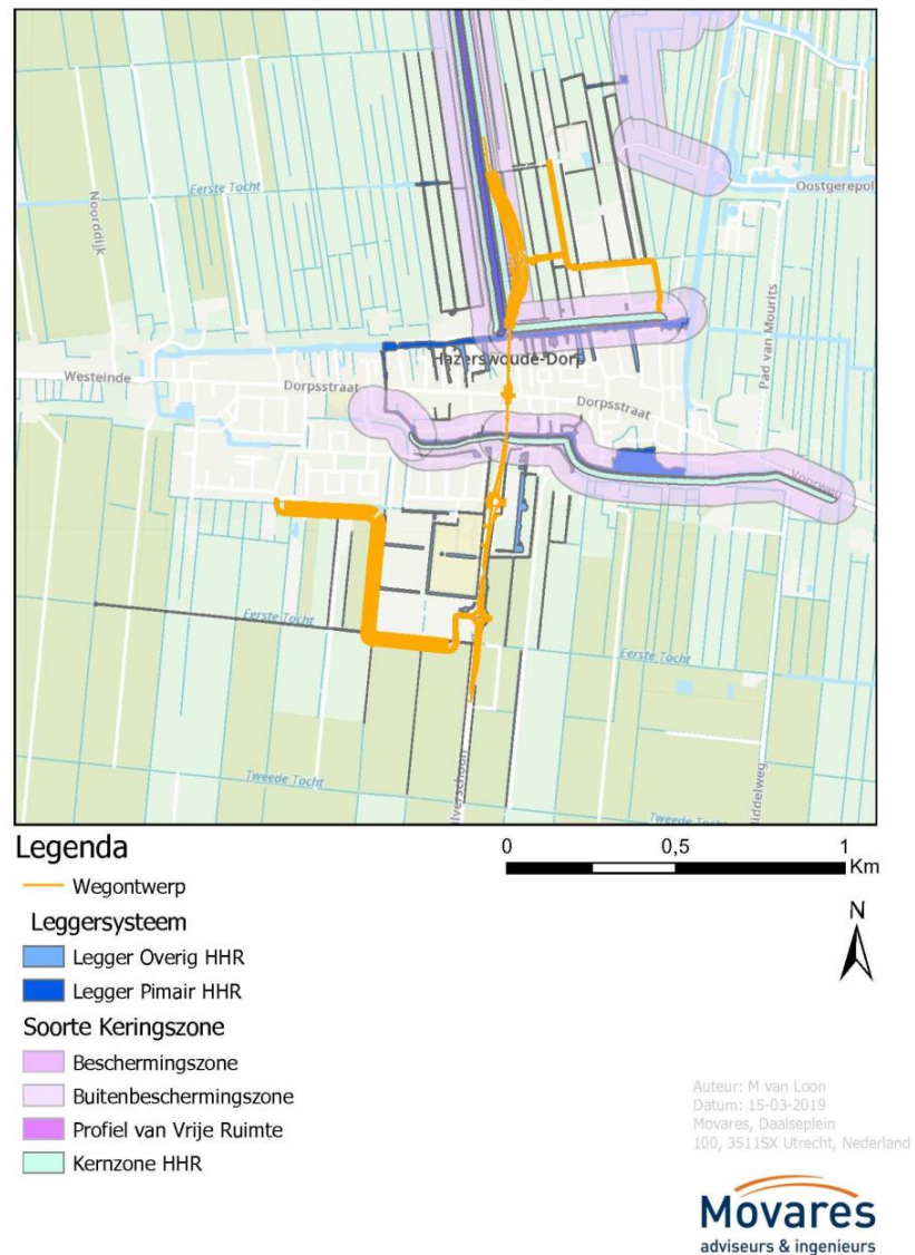
Figuur 18: regionale waterkeringen in Hazerswoude-Dorp
