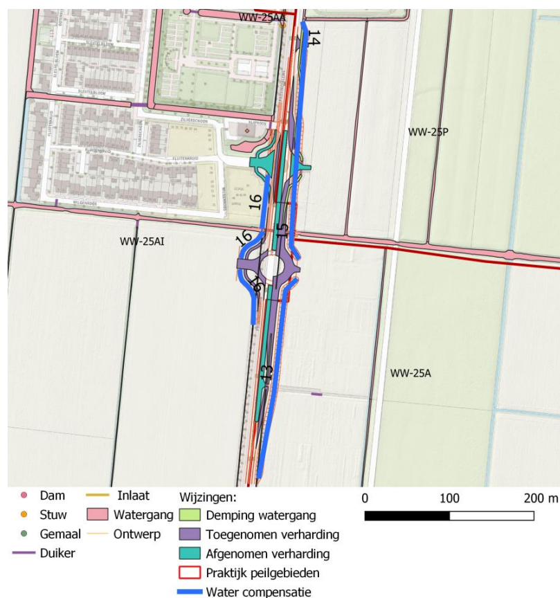
Figuur 26: Maatregelenpakket N207 Zuid met noord-west afslag N209-Dorpsstraat, overzicht verharding en watergangen aanpassingen peilvakken WW25-AI, WW25-A, WW25-P
