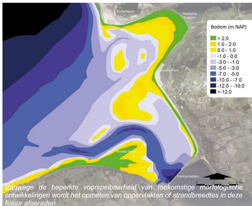
Figuur 64: Mogelijk toekomstige bodem anno 2030 - Scenario 1
