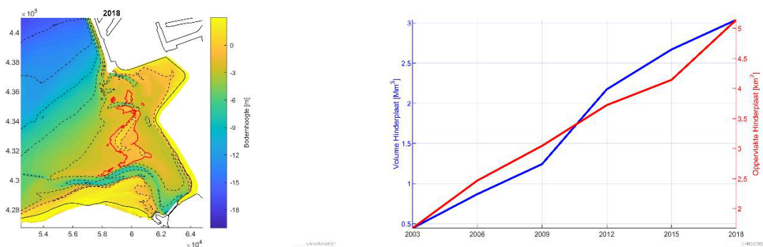
Figuur 26: Veranderingen inhoud en oppervlakte Hinderplaat 2003-2018
