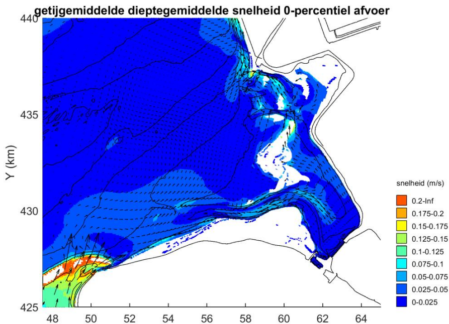
Figuur 14: Getijgemiddelde dieptegemiddelde snelheden - 2018
