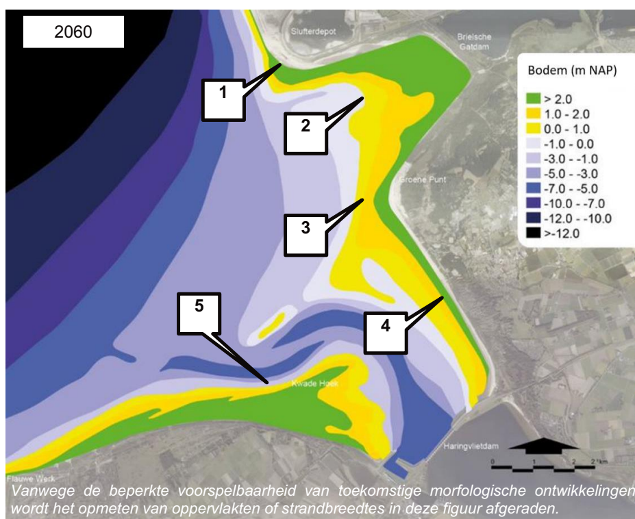
Figuur 96: Mogelijke toekomstige bodem anno 2060 voor scenario 1.
