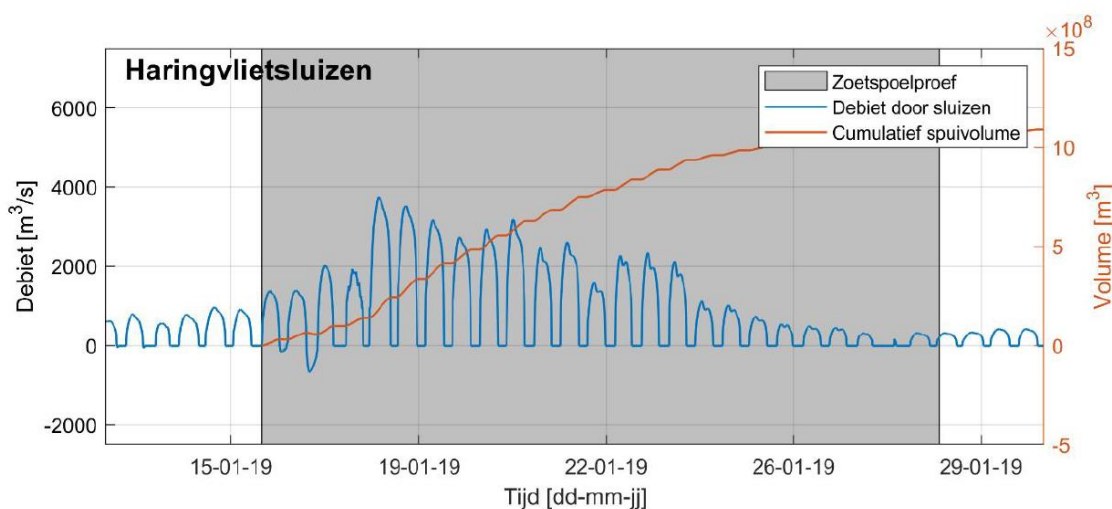
Figuur 80: Debiet door spuisluizen tijdens Kier-variant proef januari 2019 (Deltares, 2019)
