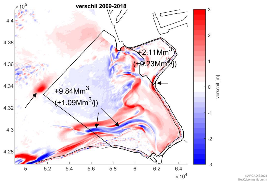
Figuur 24: Erosie-sedimentatiekaart 2009-2018 (9 jaar)
