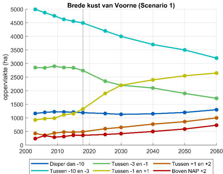
Figuur 68: Waargenomen en voorspelde veranderingen in oppervlakten van bepaalde dieptezones – scenario 1
