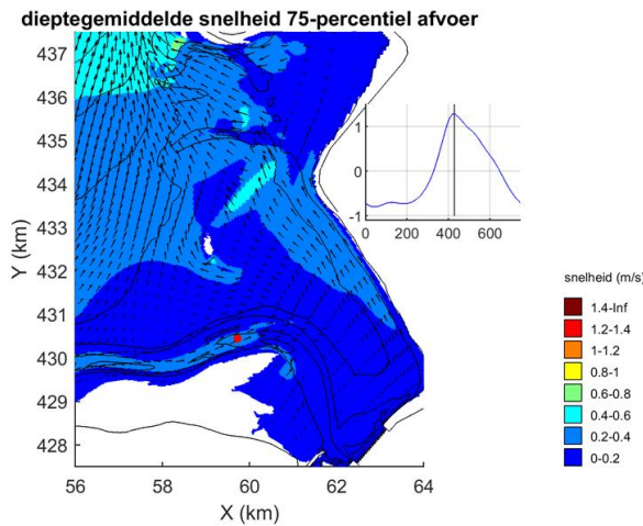
Figuur 45: Berekende diepte-gemiddelde stromingsvectoren
