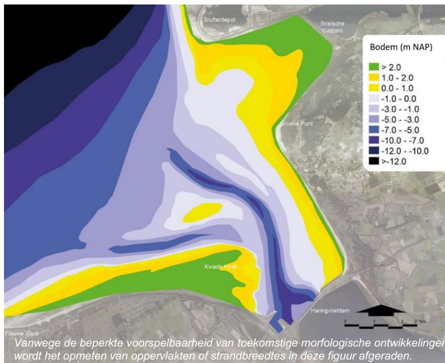
Figuur 75: Mogelijk toekomstige bodem anno 2060 - Scenario 3
