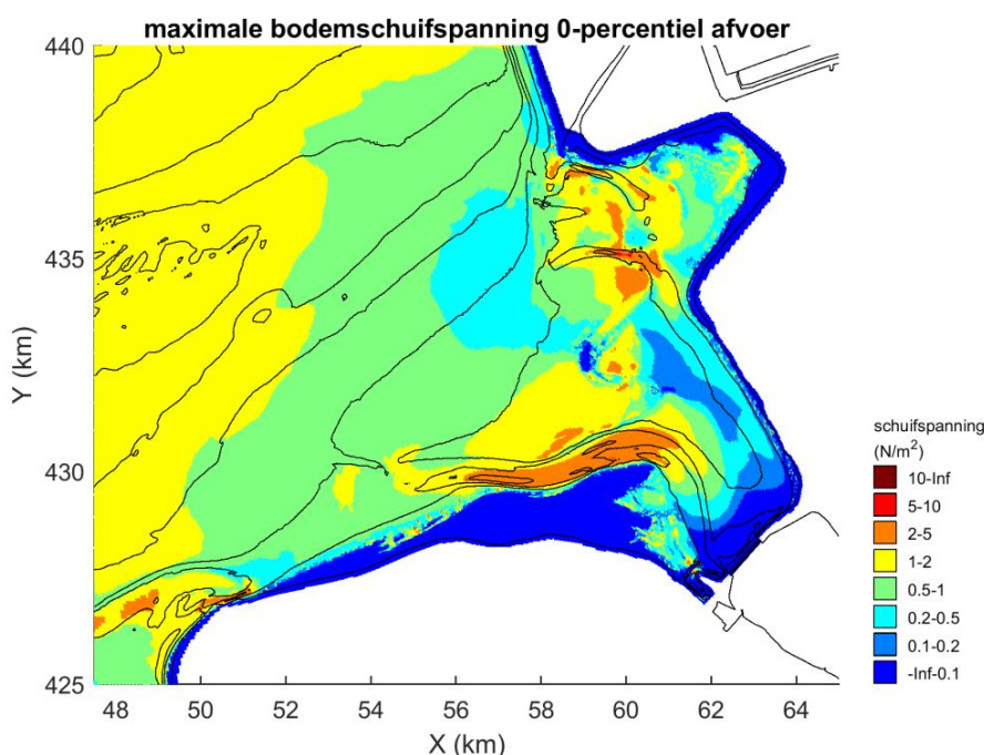
Figuur 18: Maximale bodemschuifspanning over de getijdecyclus (geen rivierafvoer)
