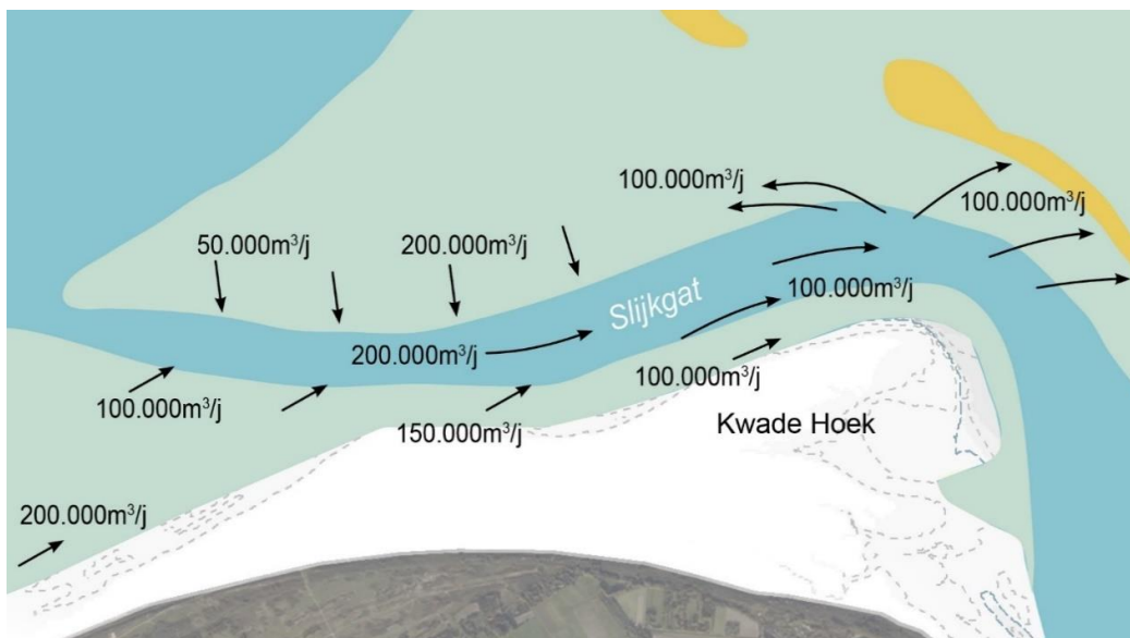
Figuur 56: Mogelijk maatgevende sedimenttransporten – Slikgat
