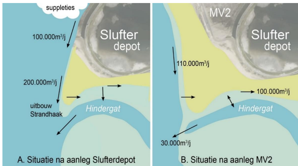
Figuur 41: Mogelijk maatgevende sedimenttransporten – gebied rondom Hindergat. A: Situatie na aanleg Sluftekdijk; B: Situatie na aanleg MV2
