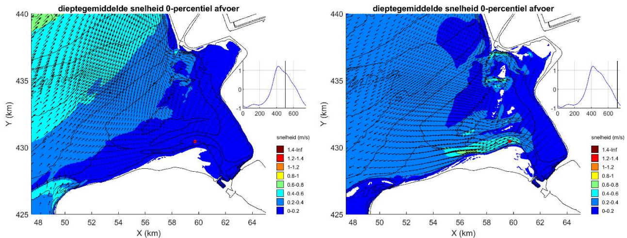
Figuur 16: Stroombeeld aan het begin van de ebperiode (links) en aan het eind (rechts) voor 2003
