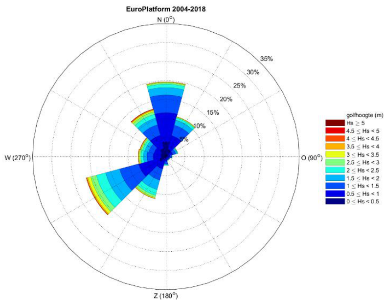
Figuur 5: Golfklimaat bij meetlocatie Europlatform
