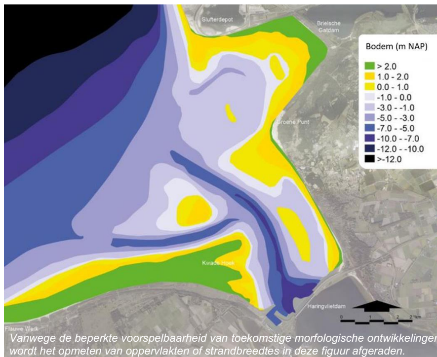
Figuur 74: Mogelijk toekomstige bodem anno 2030 - Scenario 3
