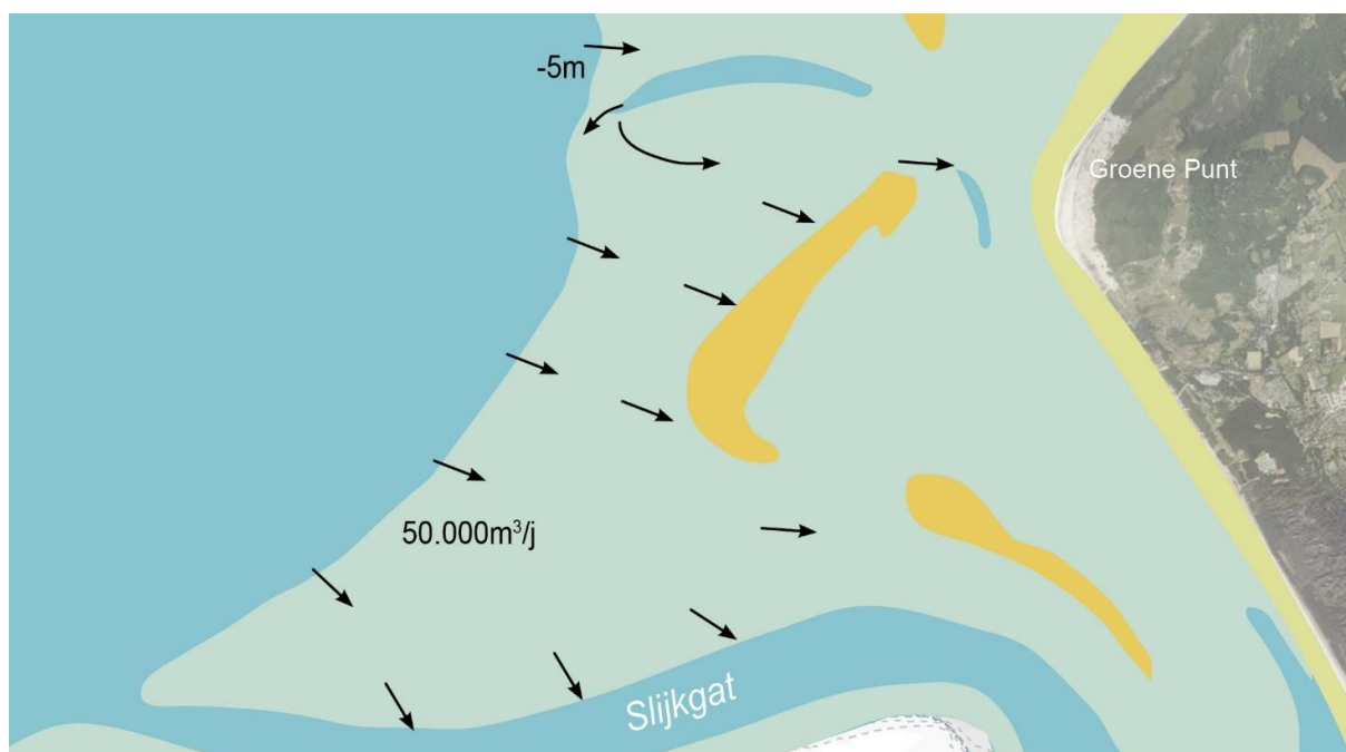
Figuur 36: Sedimentverplaatsingen vooroever
