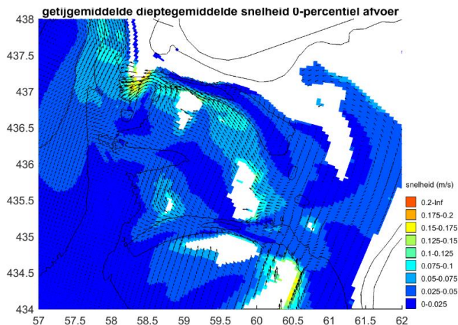
Figuur 40: Getijgemiddelde stroming Hindergat en naamloze geul
