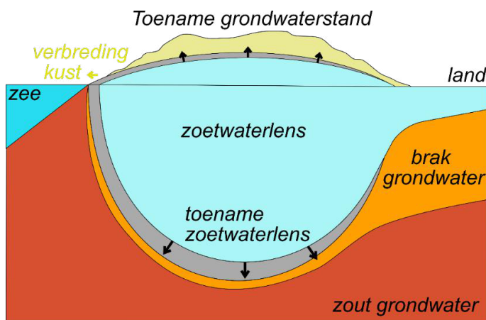
Figuur 108: Schematische weergave van een groeiende zoetwaterlens
