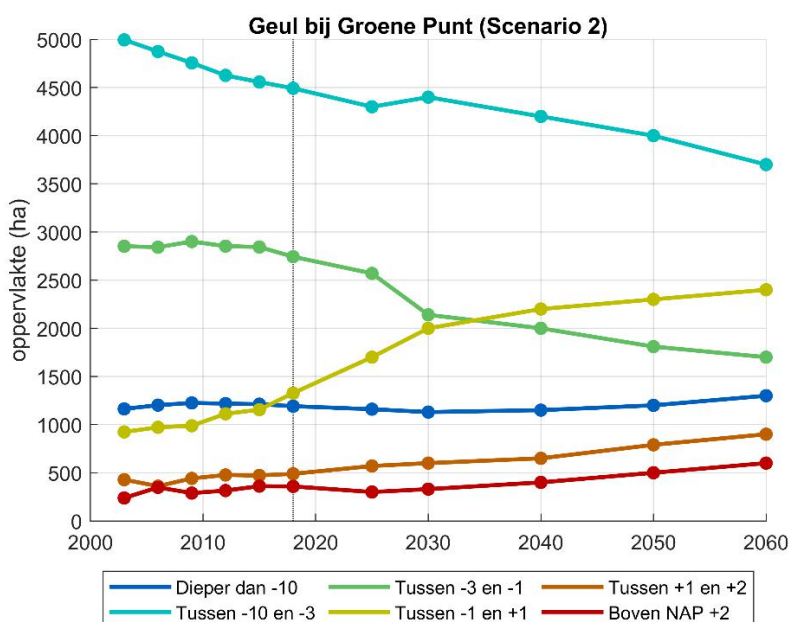
Figuur 73: Waargenomen en voorspelde veranderingen in oppervlakten van bepaalde dieptezones – scenario 2
