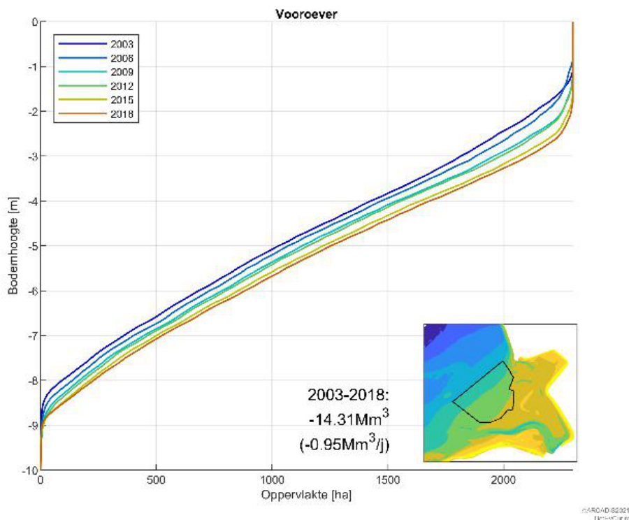
Figuur 33: Hypsometrische curves van de vooroever
