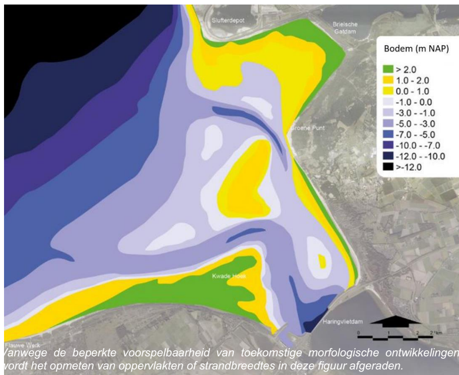
Figuur 70: Mogelijk toekomstige bodem anno 2030 - Scenario 2
