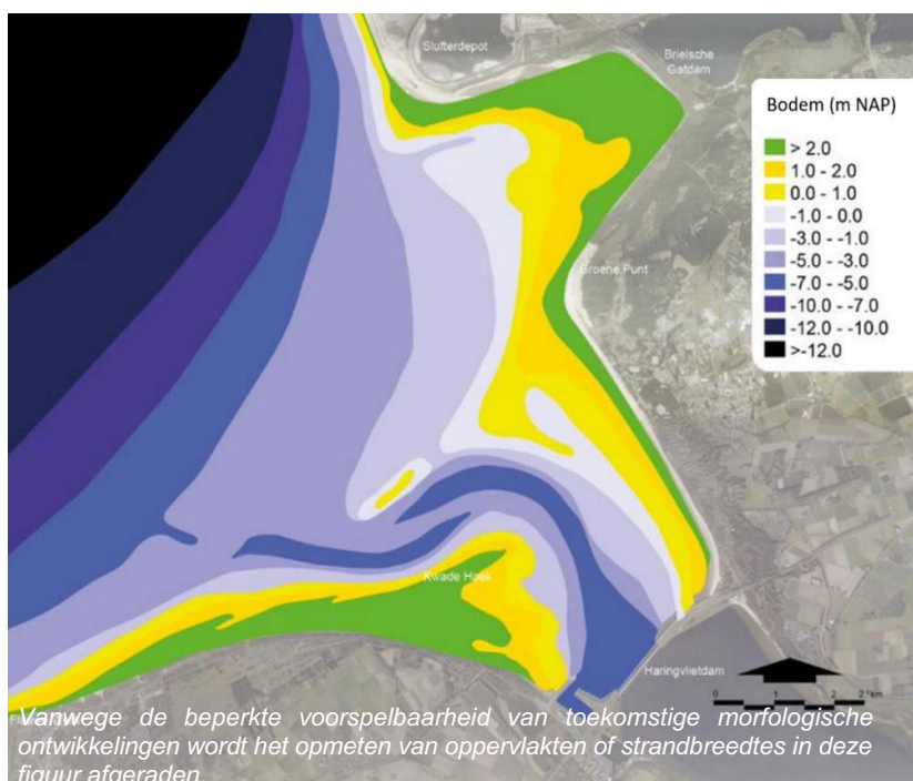
Figuur 65: Mogelijk toekomstige bodem anno 2060 - Scenario 1
