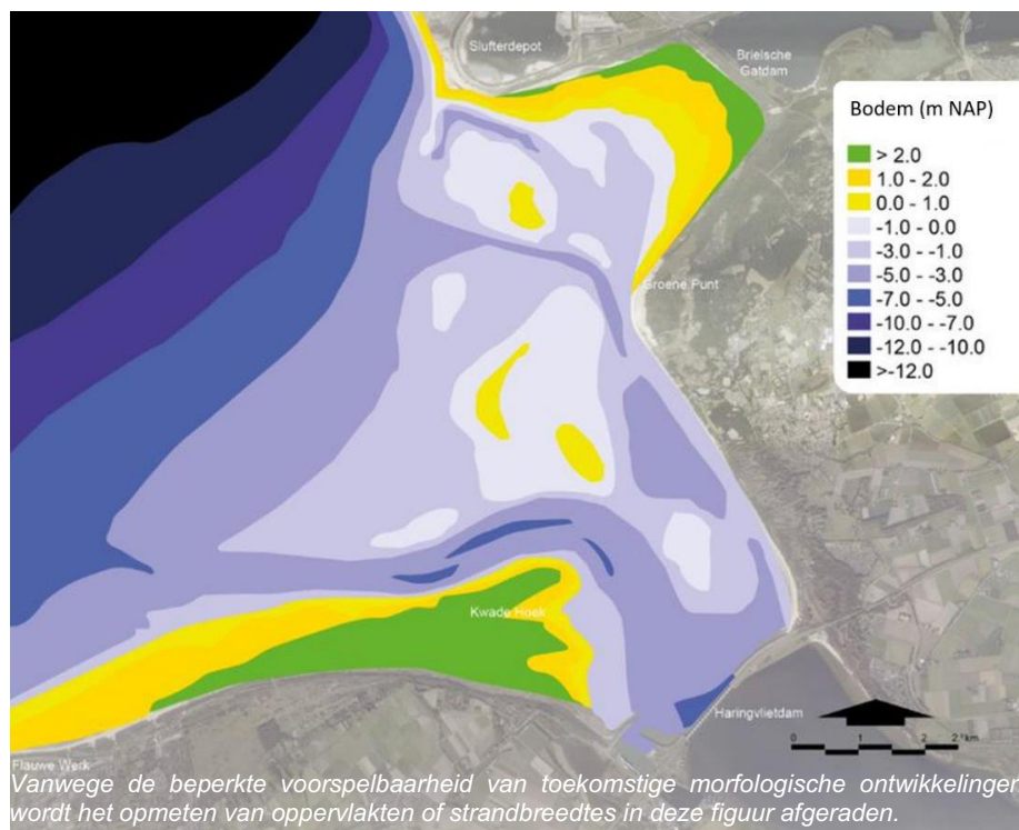
Figuur 69: Mogelijk toekomstige bodem anno 2025 - Scenario 2
