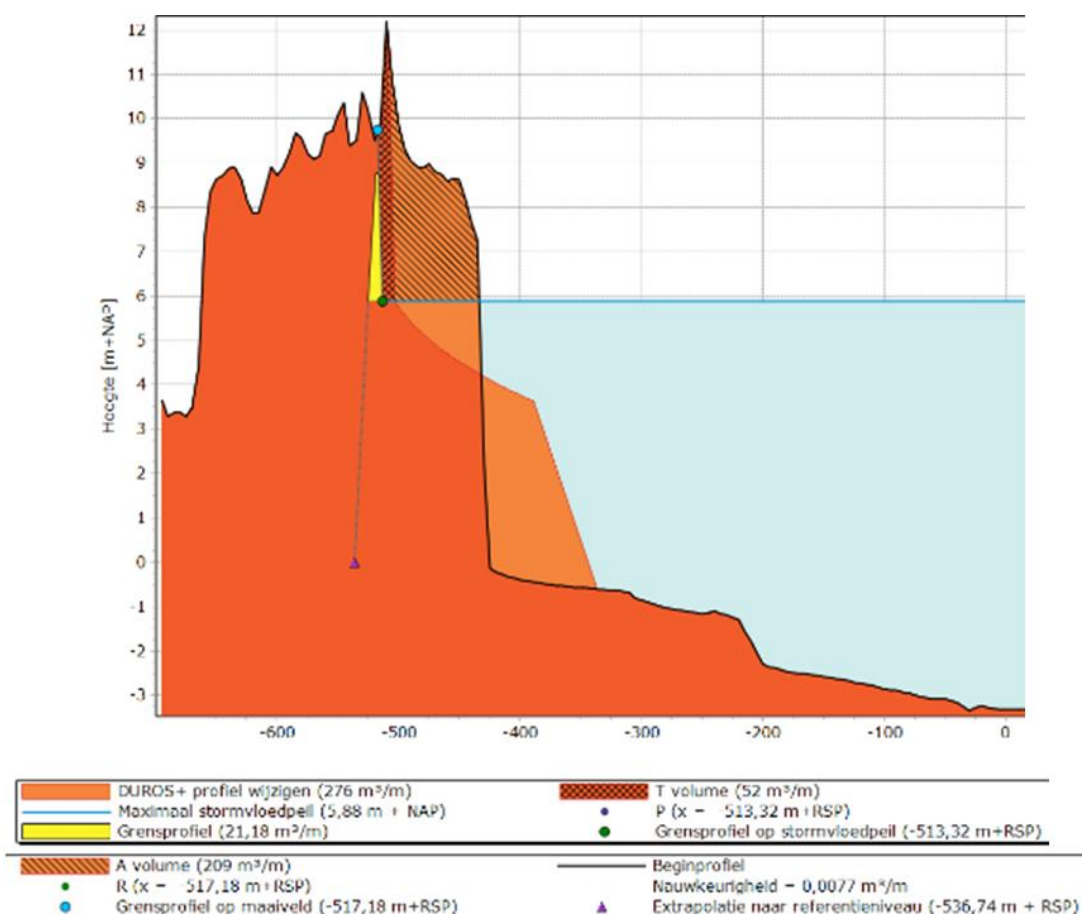
Figuur 87: Berekend afslagprofiel - referentie situatie 2031
