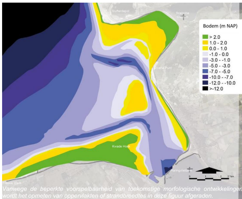
Figuur 71: Mogelijk toekomstige bodem anno 2060 - Scenario 2
