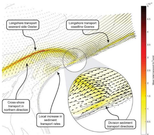
Figuur G: Gemiddelde gesimuleerde sedimenttransport na een getijdecyclus voor een laag scenario. (Groenewegen, 2019)
