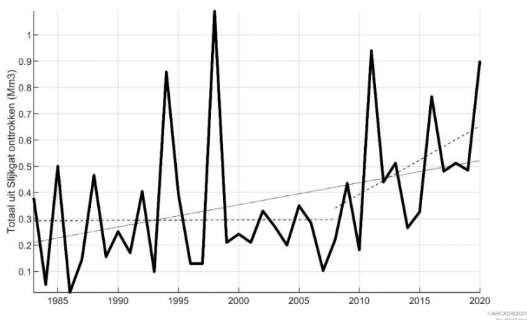
Figuur 3: Baggervolumes Slijkgat 1983-2020
