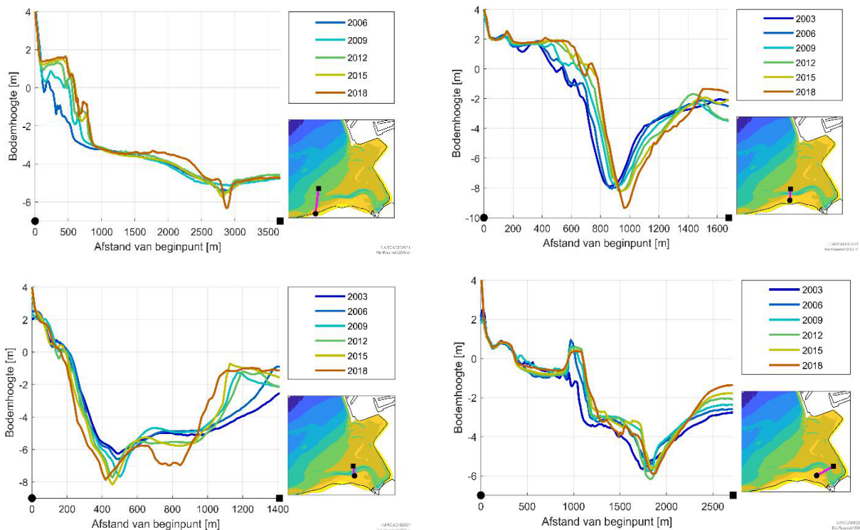
Figuur 30: Dwarsprofielen op vier locaties dwars op het Slikgat (en kust van Goeree)
