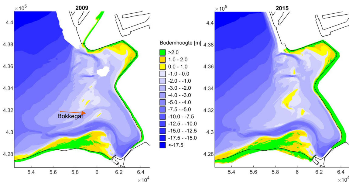
Figuur 25: Bodemligging 2009 (links) en 2015 (rechts)
