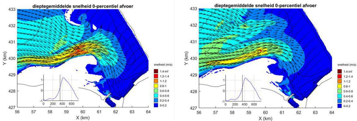
Figuur 51: Vloedstroming (geen rivierafvoer) bij Kwade Hoek 2018 (links) en 2003 (rechts)
