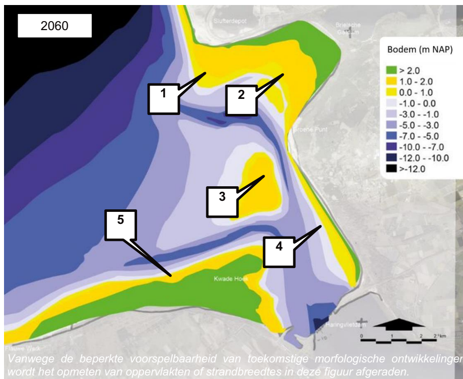
Figuur 97: Mogelijke toekomstige bodem anno 2060 voor scenario 2.
