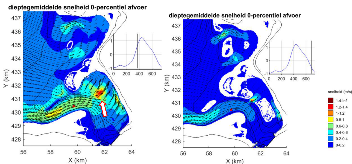
Figuur 67: Berekende stroomsnelheden 2030: links vloedstroom, rechts ebstroom
