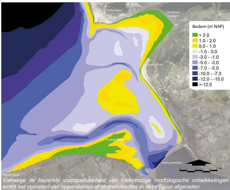
Figuur 63: Mogelijk toekomstige bodem anno 2025 - Scenario 1
