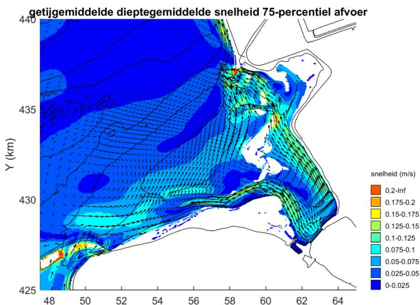
Figuur 21: Getijgemiddelde dieptegemiddelde snelheden
