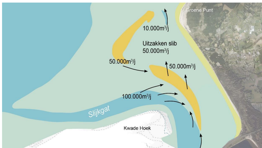
Figuur 52: Mogelijk maatgevende sedimenttransporten – vooroever kust van Voorne
