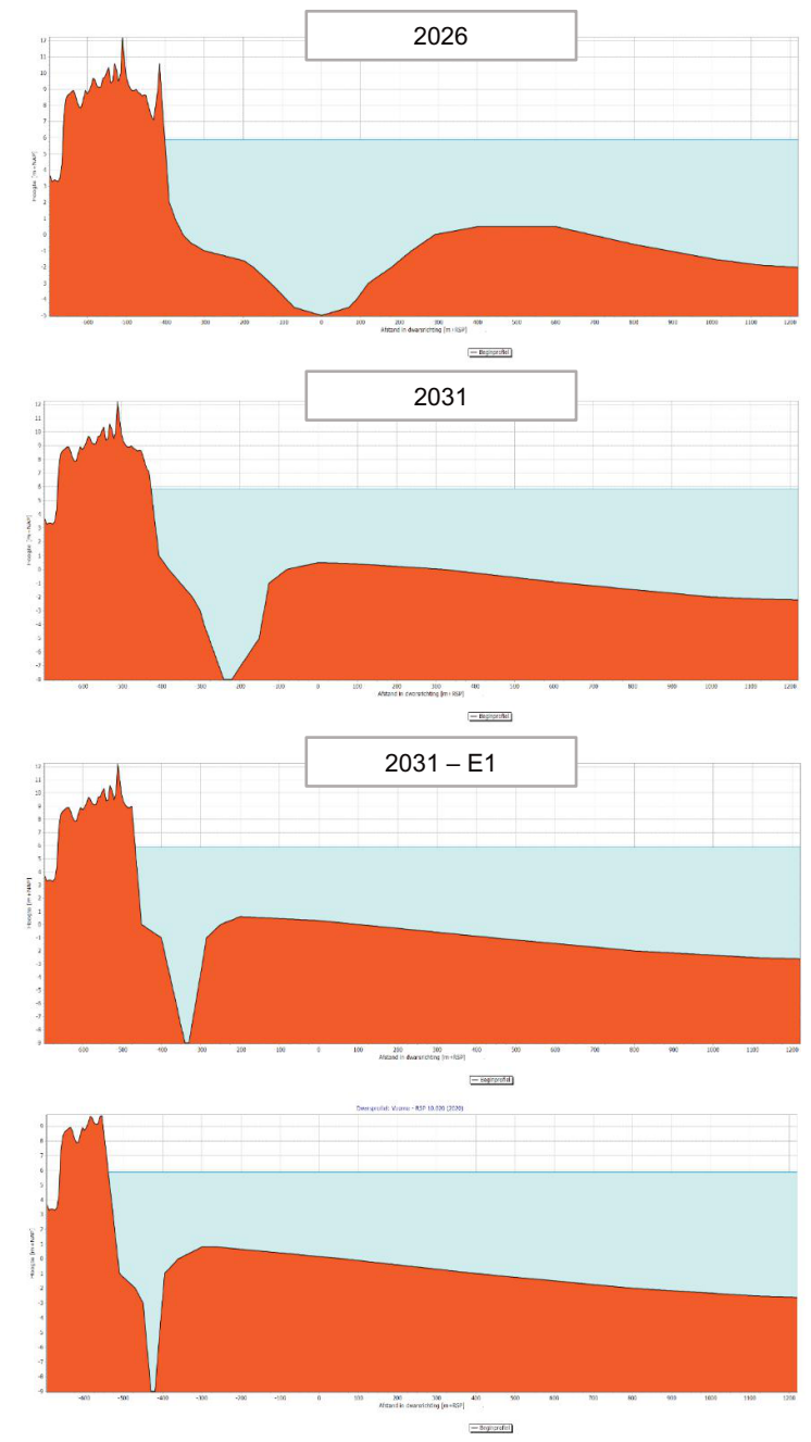
Figuur 83: Mogelijke toekomstige veranderingen in kustprofiel RSP 10.020 (Voorne) voor 2020, 2026 en 2031. Voor 2031 zijn er twee extreme situaties: 'E1' en 'E2'.
