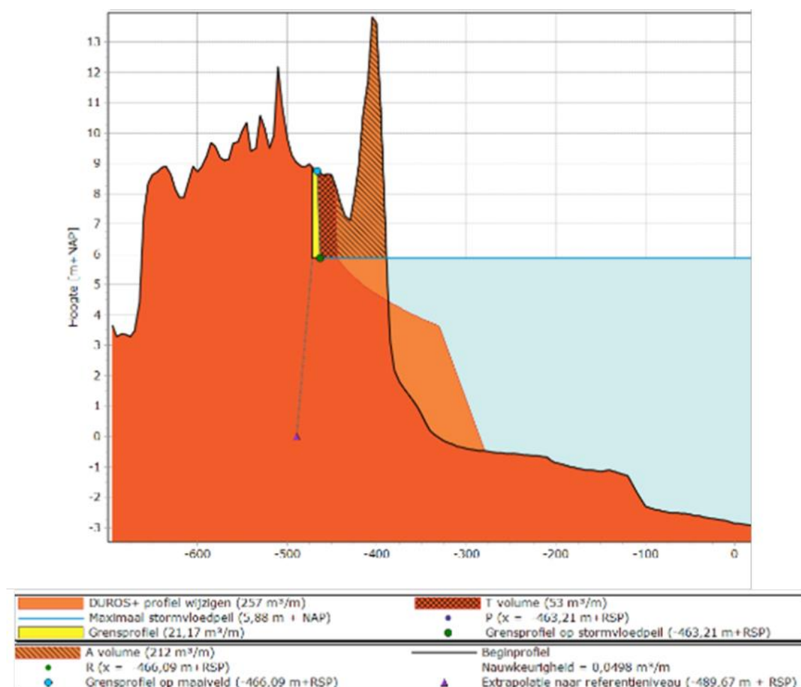
Figuur 86: Berekend afslagprofiel - huidige situatie 2020
