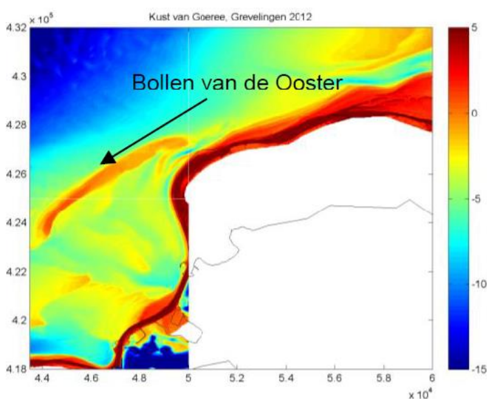
Figuur 79: Morfologie mondingsgebied Grevelingen anno 2012
