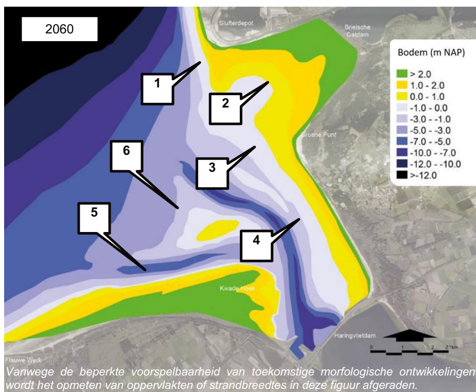
Figuur 98: Mogelijke toekomstige bodem anno 2060 voor scenario 3.
