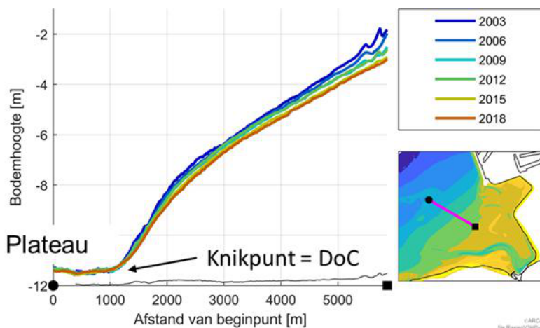
Figuur 35: actieve deel van de vooroever (profielen 2003 – 2018)
