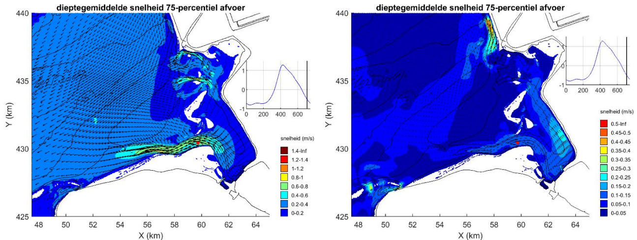
Figuur 20: Stroombeeld aan het begin van de ebperiode (links) en netto-effect spuidebiet (rechts)
