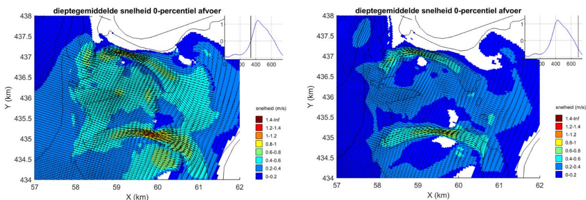
Figuur 39: Maximale vloedstroming (links) en maximale ebstroming (rechts) Hindergat en naamloze geul
