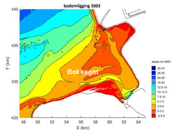
Figuur 5 Samengestelde modelbodem voor 2003 met Bokkegat
