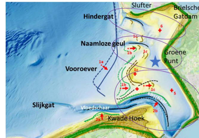
Figuur 7 Weergave van persistente morfologische veranderingen
