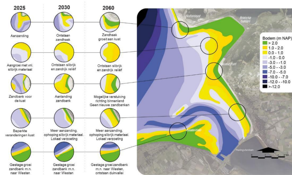
Figuur 12 Morfologische ontwikkelingen en dieptezones voor 2025, 2030 en 2060.
