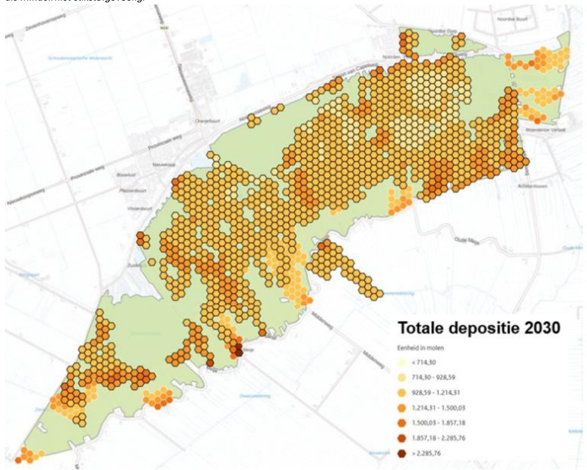
Figuur 8-3. Berekende depositiewaarden in 2030 in Natura 2000-gebied Nieuwkoopse Plassen & De Haek. De wit omlijnde hexagonen zijn locaties waar H6430A of H6430B ligt. Deze habitattypen hebben een KDW >2400 en zijn door Wamelink et al., (2023) zijn beoordeeld als minder/niet stikstofgevoelig.
