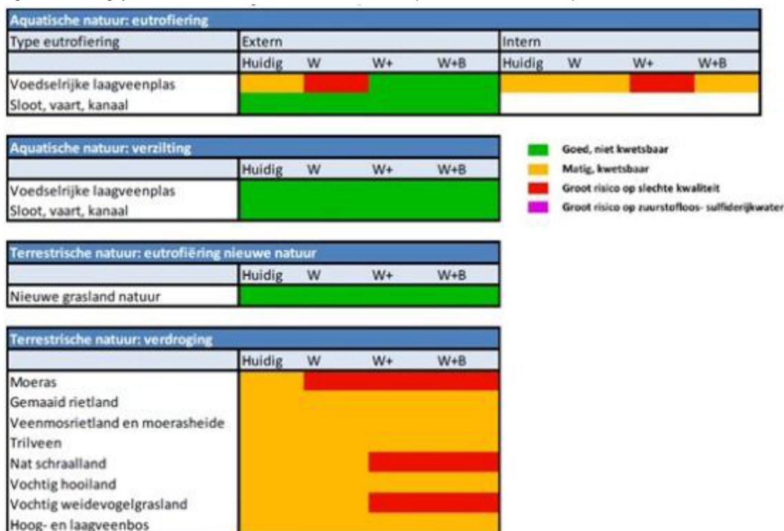
Figuur 6-5. Belangrijkste resultaten klimaatscenario studie Nieuwkoopse Plassen & De Haack op basis van de KNMI'06-scenario's
