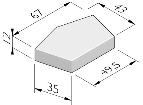
Steen voor het duinplein: Penta 43x67 van Struyk Verwo Infra. In de zandkleur Lavarogel/bruin 440.
