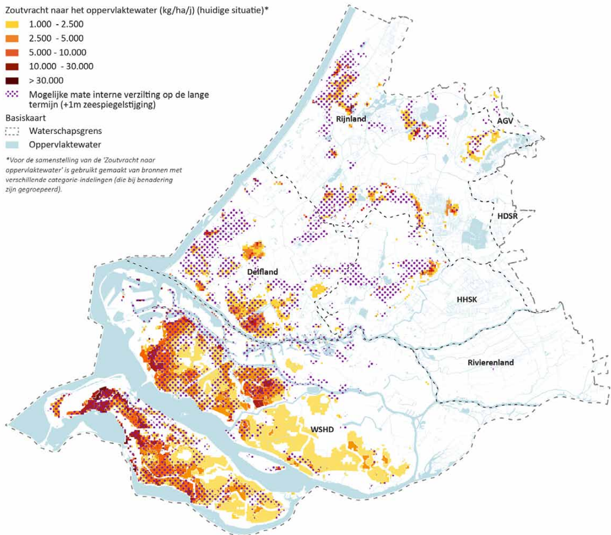
FIG. A.3.11 Kaart zoutvracht naar oppervlaktewater, bij voldoende zoetwaterbeschikbaarheid voor doorspoeling betekent dit niet dat het zout wat zich ook daadwerkelijk in het oppervlaktewater bevindt. (kaart: Defacto, bron data: Deltares 2022, Rijkswaterstaat, Deltares, Arcadis, Hydrologic, Ministerie van Infrastructuur en Waterstaat, 2024; aangevuld met data van WSHD van de verzilting op Goeree, Voorne Putten en Hoeksche Waard).
