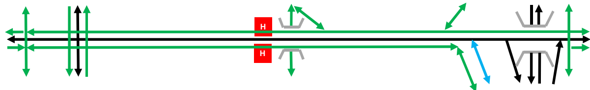
Variant 5: Nota Voorkeursmaatregelen gewijzigd + oversteek bij kruispunt Raadhuis
