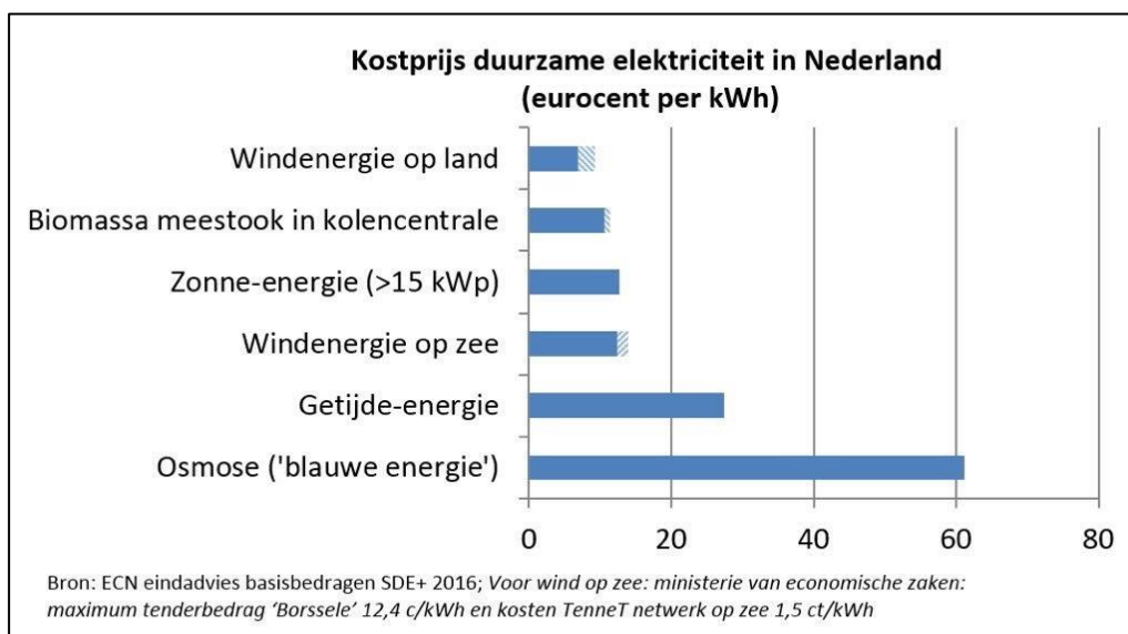
Figuur 2.1 Kostprijs duurzame elektriciteit in Nederland
