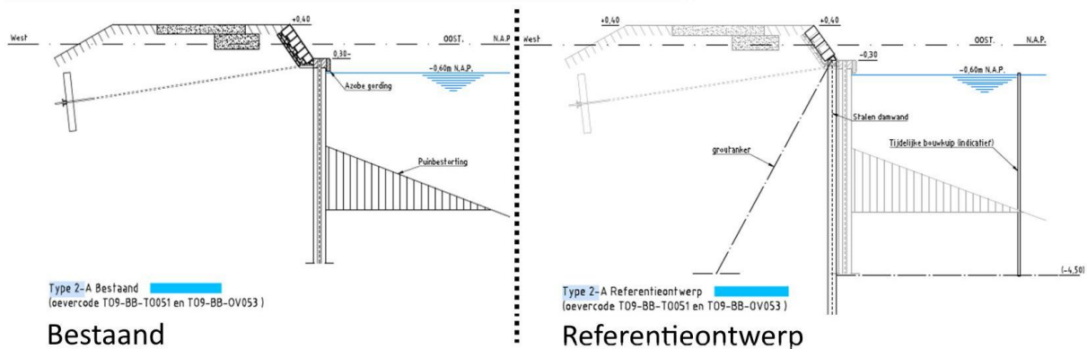
Figuur 3-2: Oevertype vak 7. Links onder: Bestaande oeverconstructie. Rechts onder: Referentieontwerp van de oeverconstructie
