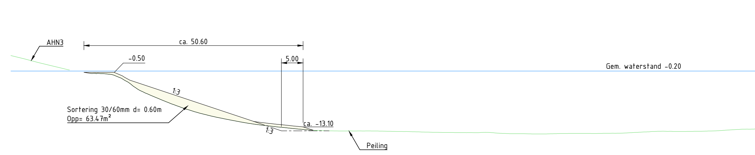
Dwarsprofiel DP-1 Schaal 1:500
