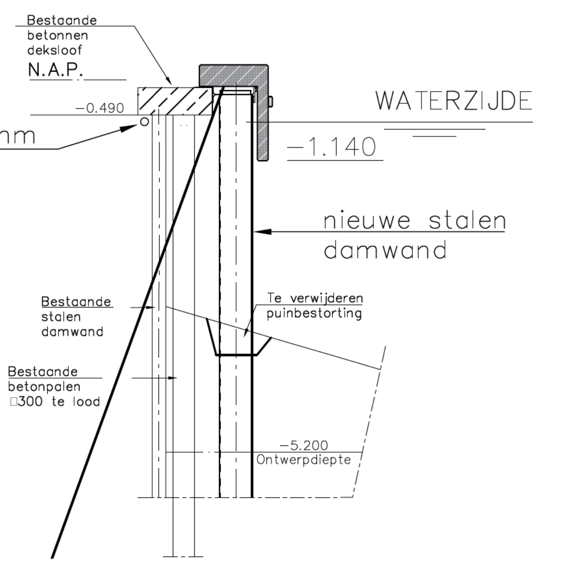
PRINCIPE DOORSNEDEN 8B SCHAAL 1:50
