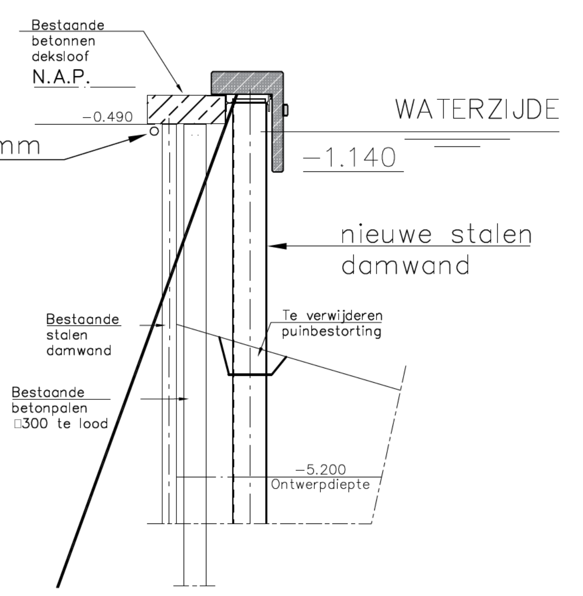
PRINCIPE DOORSNEDE 8B SCHAAL 50
