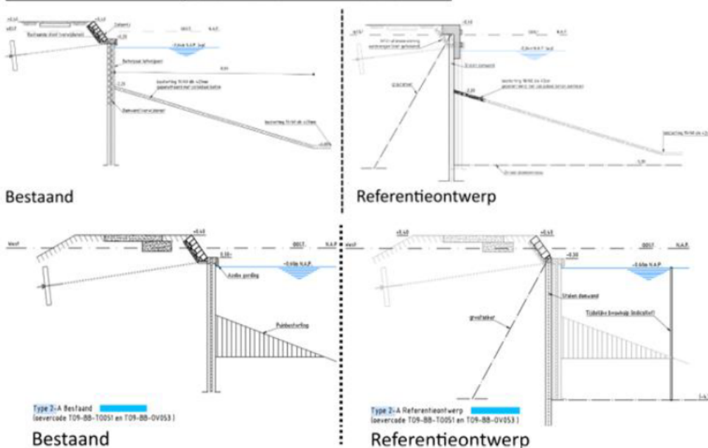
Figuur 2-2: Ontwerp oevertype 4 en huidige en voorgenomen oeverconstructie
