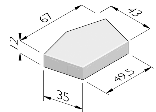
Steen voor het duinplein: Penta 43x67 van Struyk Verwo Infra. In de zandkleur Lavaro geel/bruin 440.
