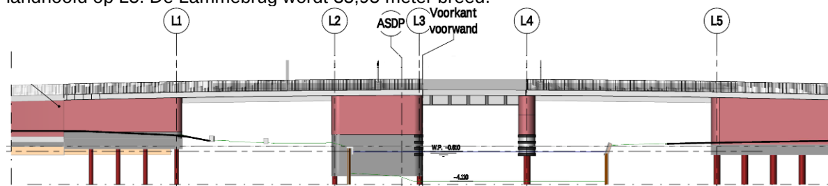
FIGUUR 2 – LANGSAANZICHT LAMMEBRUG
