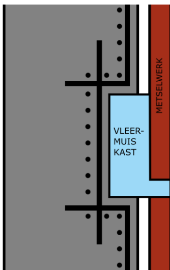
FIGUUR 14 – DOORSNEDE WAND MET GEÏNTEGREERDE VLEERMUISKAST
