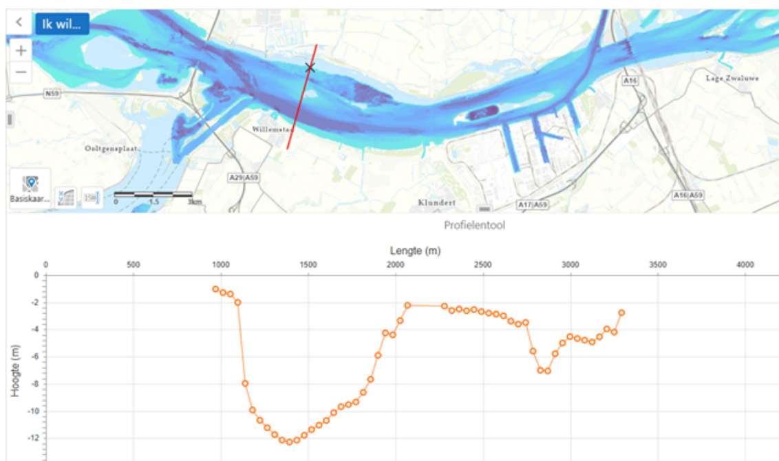
Figuur 3-17. Doorsnede van het Hollandsch Diep (west). Het profiel loopt van zuid naar noord. Bron: Rijkswaterstaat.
