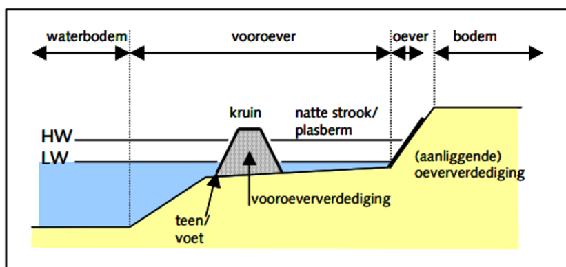
Figuur 3-25: Schematische weergave vooroeverbescherming (Gelder et al., 2003).
